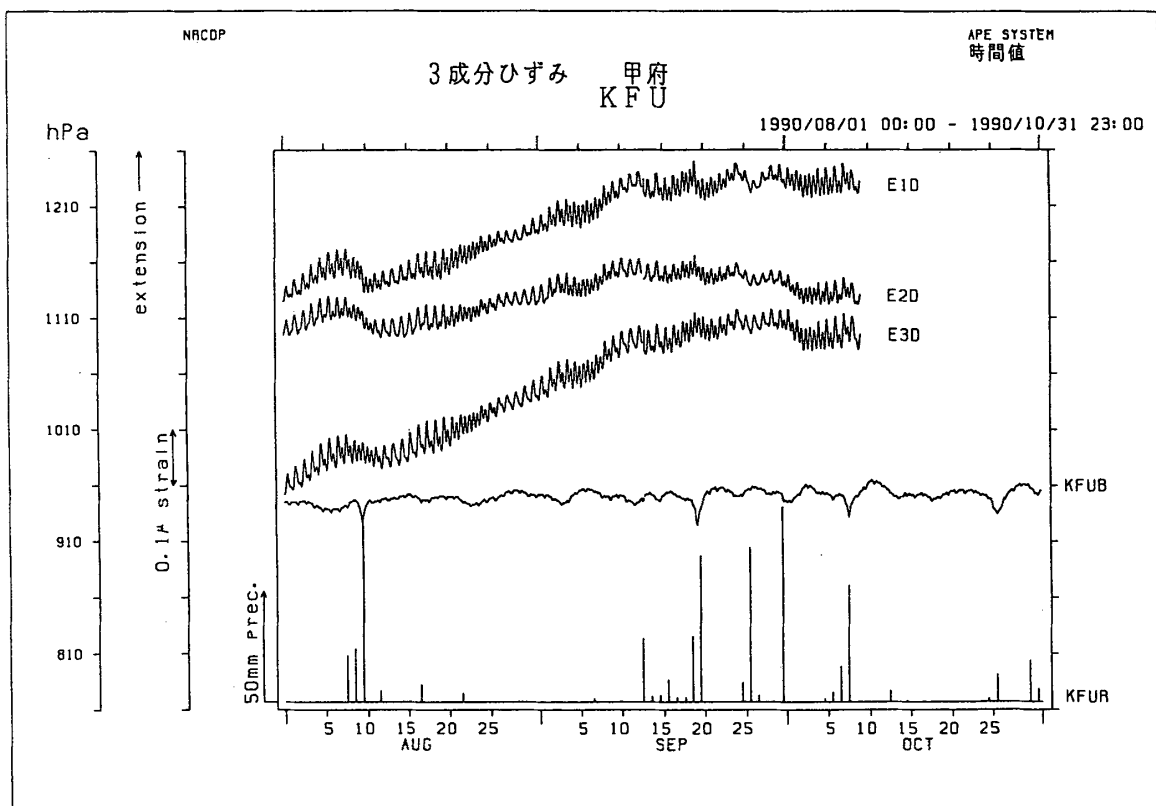
第6図 甲府観測点における時間値の観測値からドリフトを除いた残差
