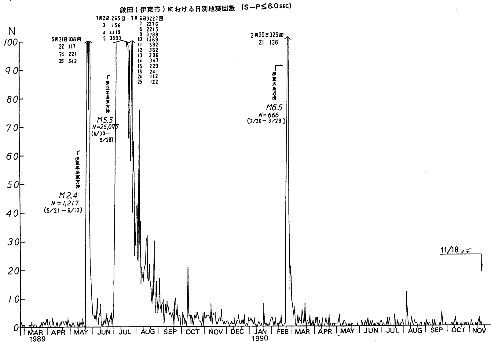
第1図 伊東市鎌田における日別地震回数 (S-P ≤ 6.0秒)
