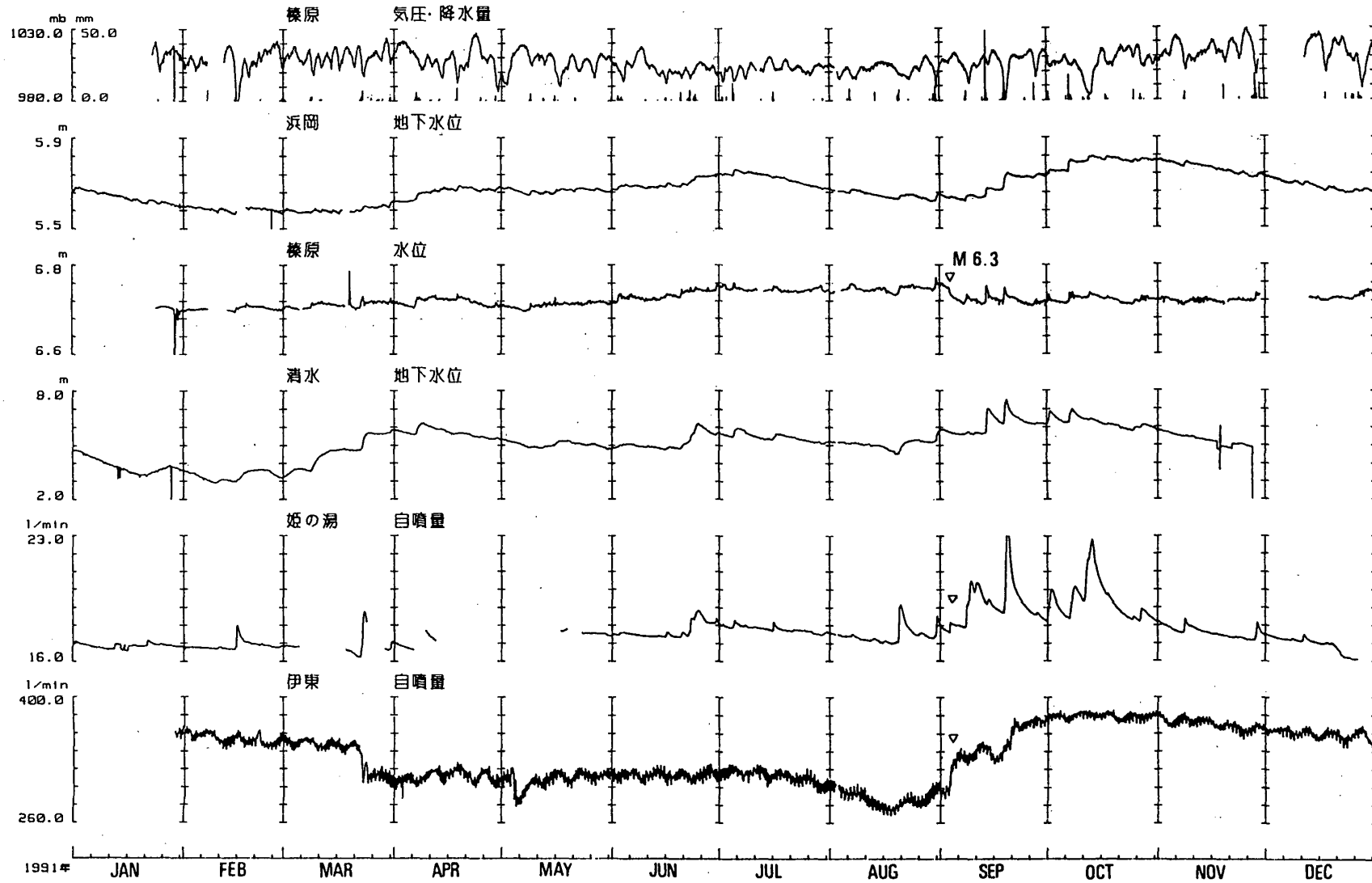
東海・伊豆地域地下水位・自噴量観測結果(1991年1月~12月,時間平均値,気圧潮汐補正)
