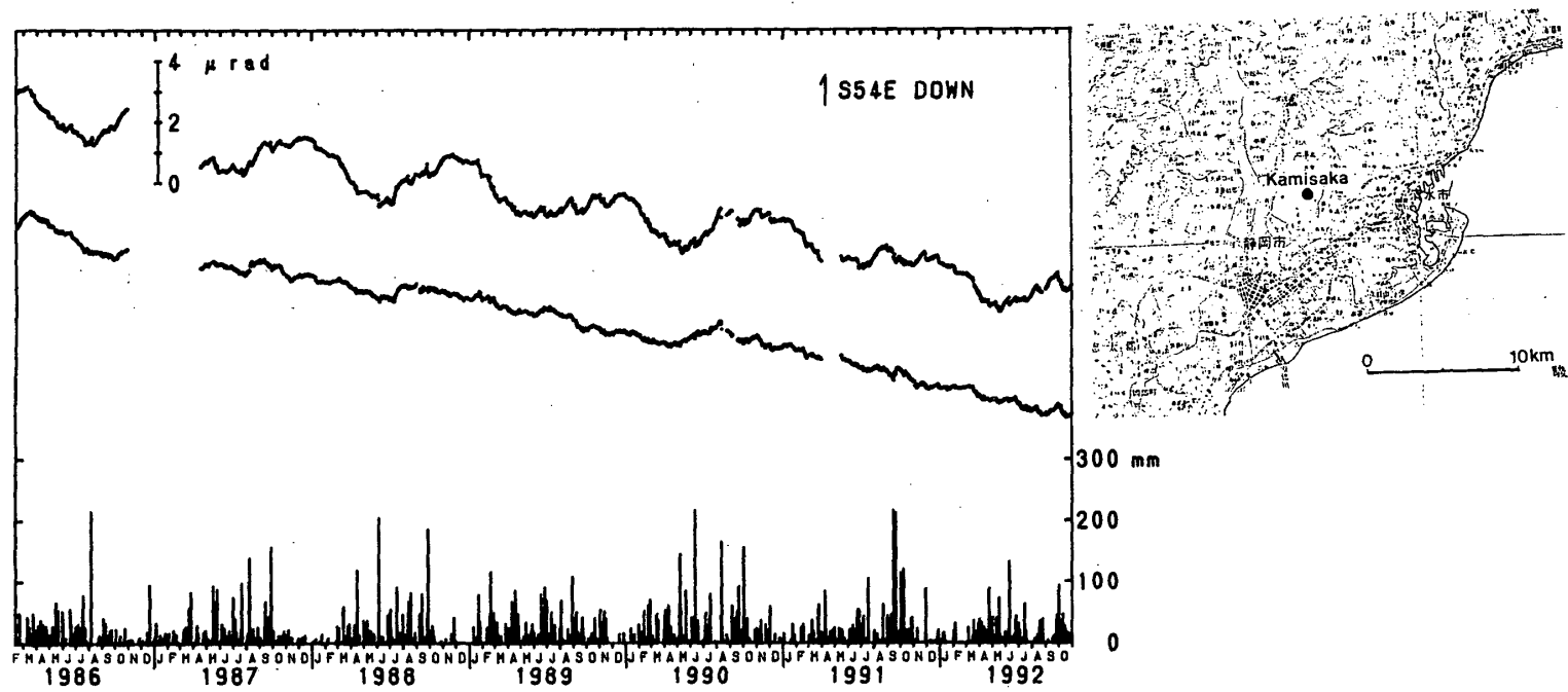
第3図 上坂観測点の水管傾斜計の日平均値と、それから年周変化と雨量の影響を取り除いた結果、および静岡地方気象台での日雨量。(1986年2月から1992年10月)
