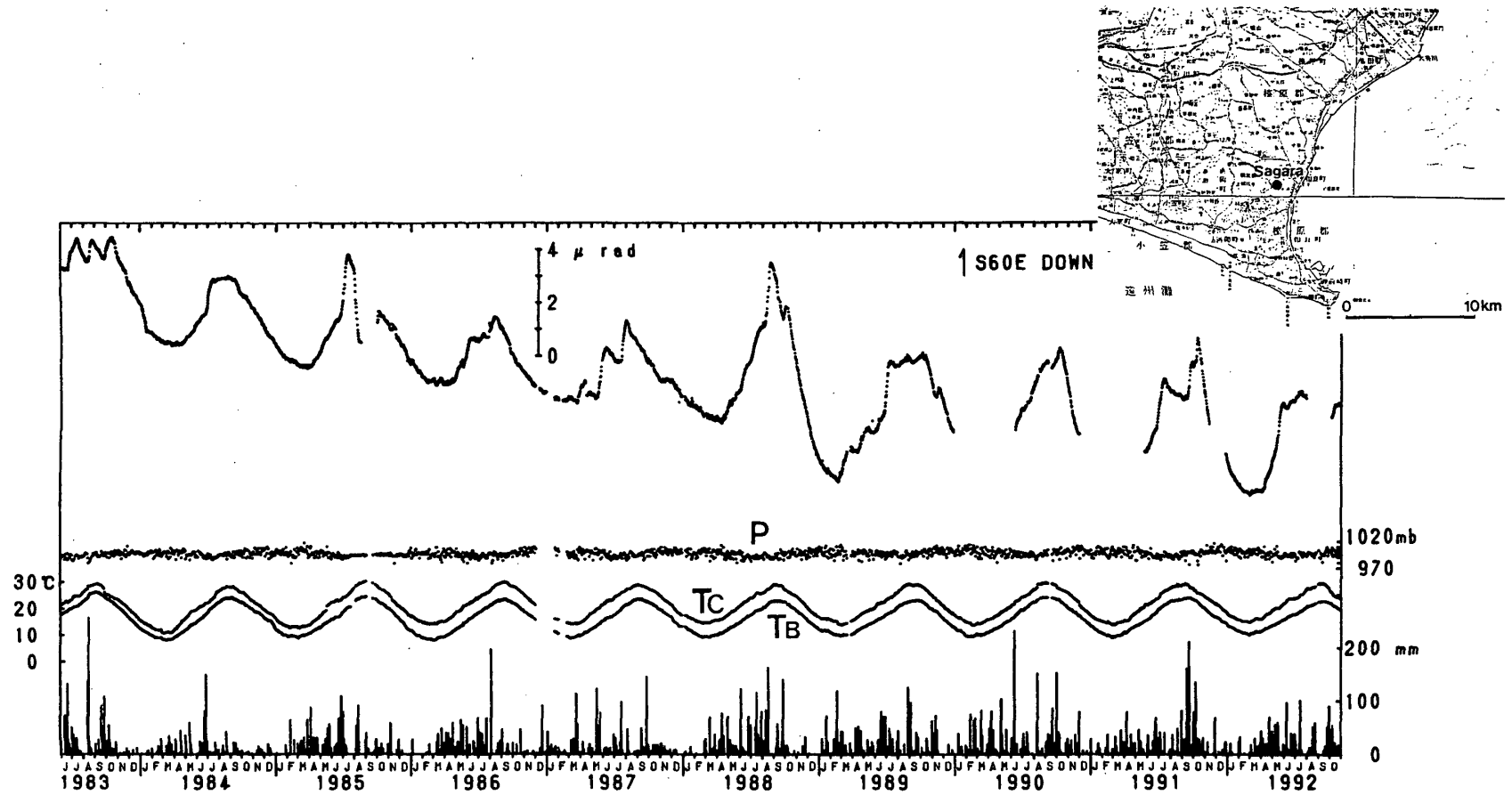
第1図 相良観測点での水管傾斜計による傾斜，気圧 (P)，傾斜計の中間点 (T c ) と北西端 (T b ) での温度の日平均値，および牧ノ原アメダスによる日雨量。(1983年6月から1992年10月)
