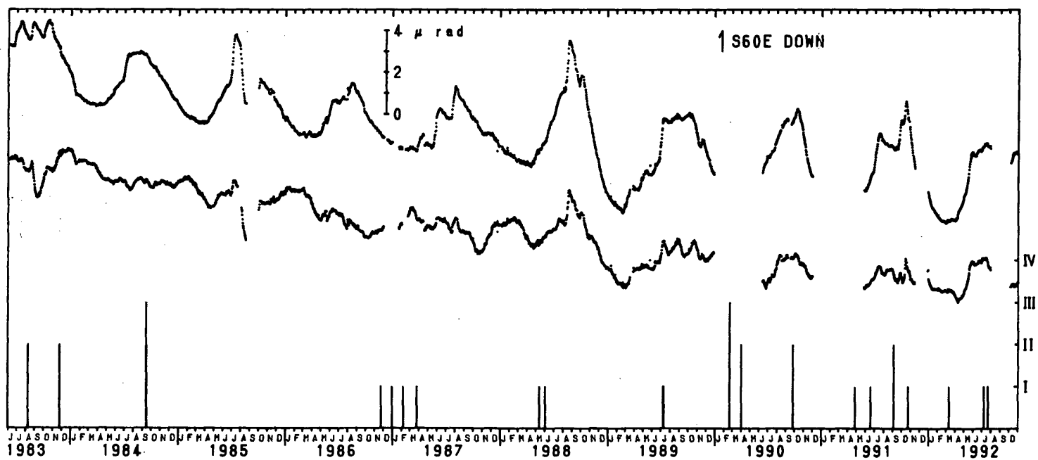
第2図 相良観測点の水管傾斜計の日平均値と、それから雨量と温度の影響を取り除いた結果。 縦線は御前崎における有感地震の震度。(1983年6月から1992年10月)
