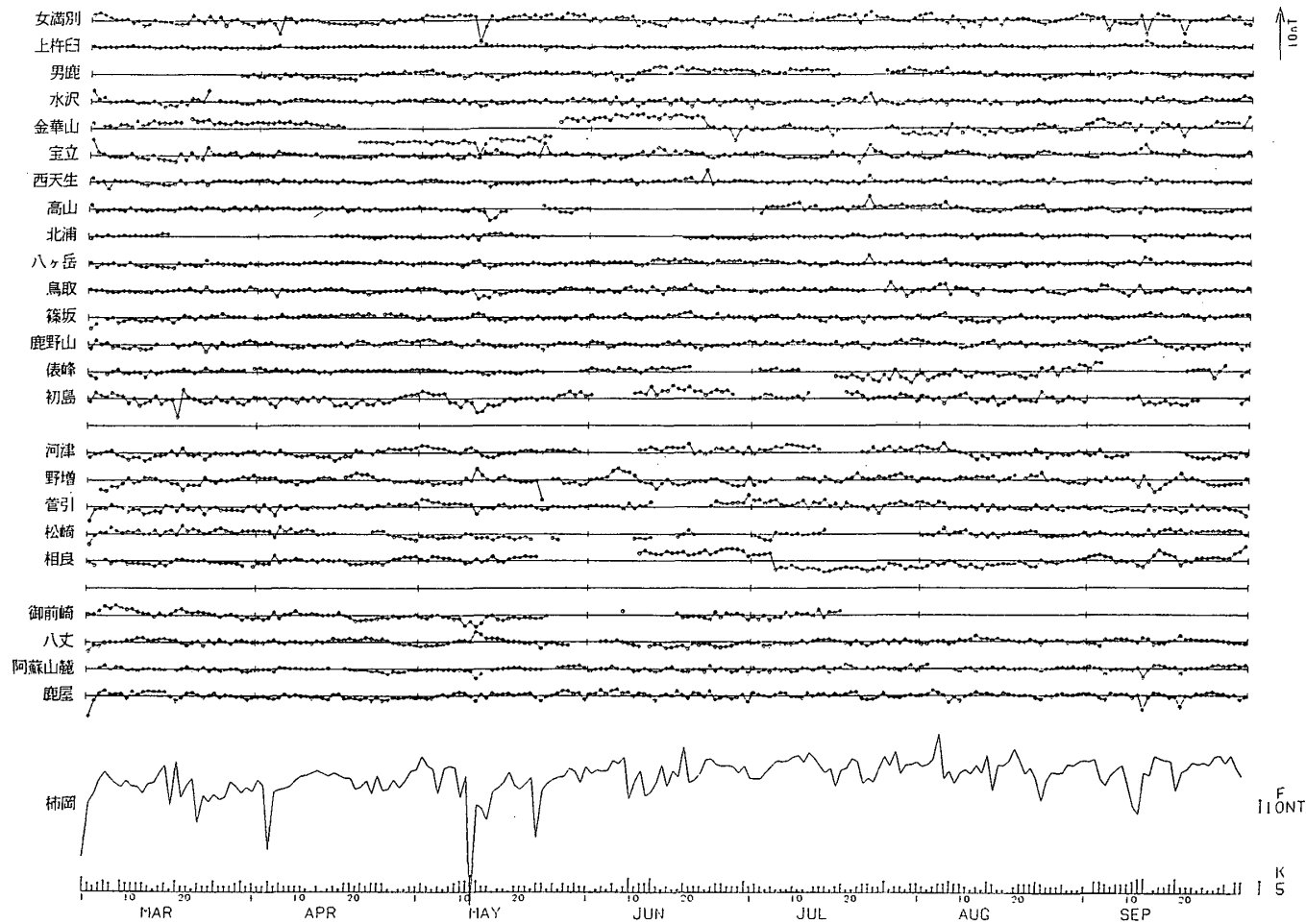
第3図 上段：拡張された主成分分析法により推定された，全磁力日平均夜間値の各観測点の局所的な変化。推定のための係数は1990年1～6月のデータに基づいて計算された。 下段：柿岡に於ける全磁力夜間値の日平均と夜間K指数。 1992年3月～1992年9月
