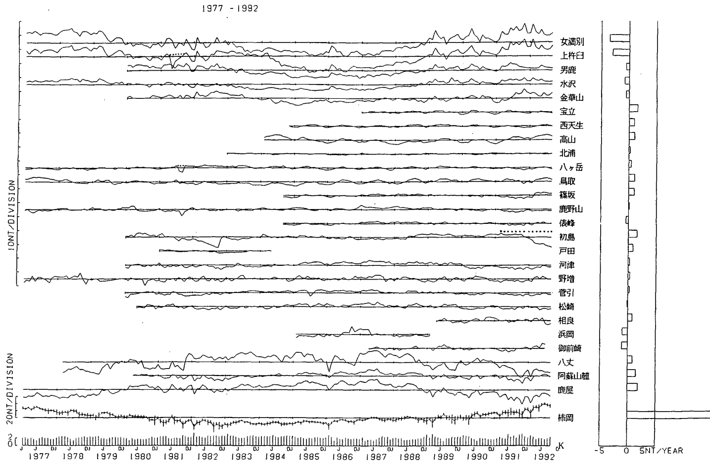
第4図 左：柿岡に対する各観測点の経年変化を除去した全磁力夜間値の単純差月平均値及び柿岡における全磁力夜間値と夜間K指数の月平均値 右：経年変化率 1977年1月～1992年9月 エラーバーは±標準偏差，点線は人工的な擾乱または測器の不調による異常値を示す。
