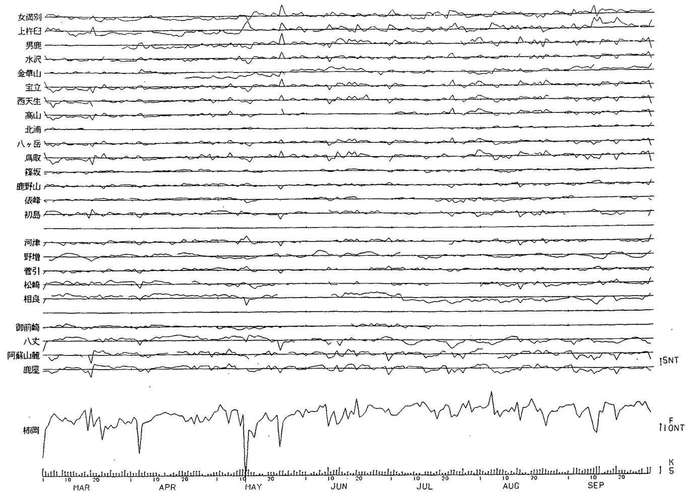
第2図 上段：柿岡に対する各観測点の全磁力夜間値の日平均値の重偏差
