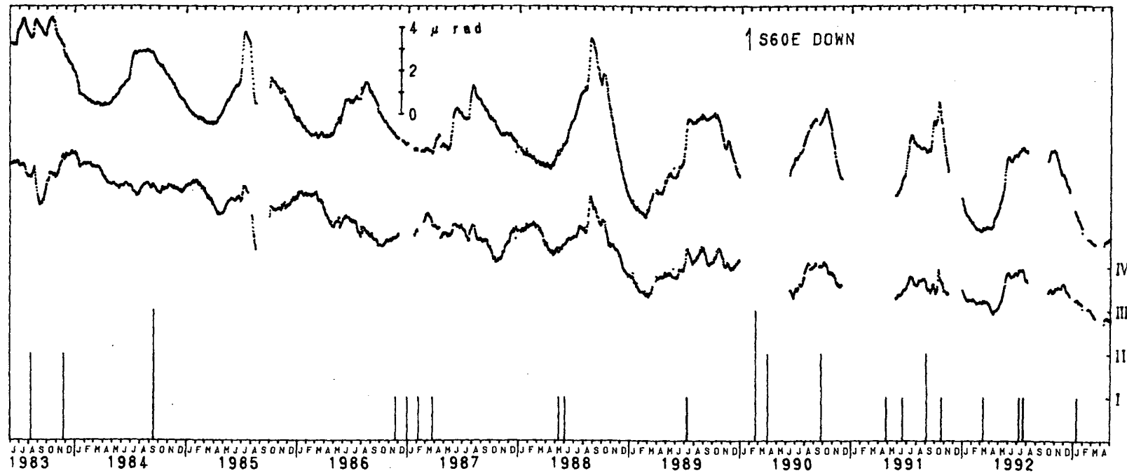
第2図 相良観測点の水管傾斜計の日平均値と、それから雨量と温度の影響を取り除いた結果。縦線は御前崎における有感地震の震度（1983年6月から1993年4月）
