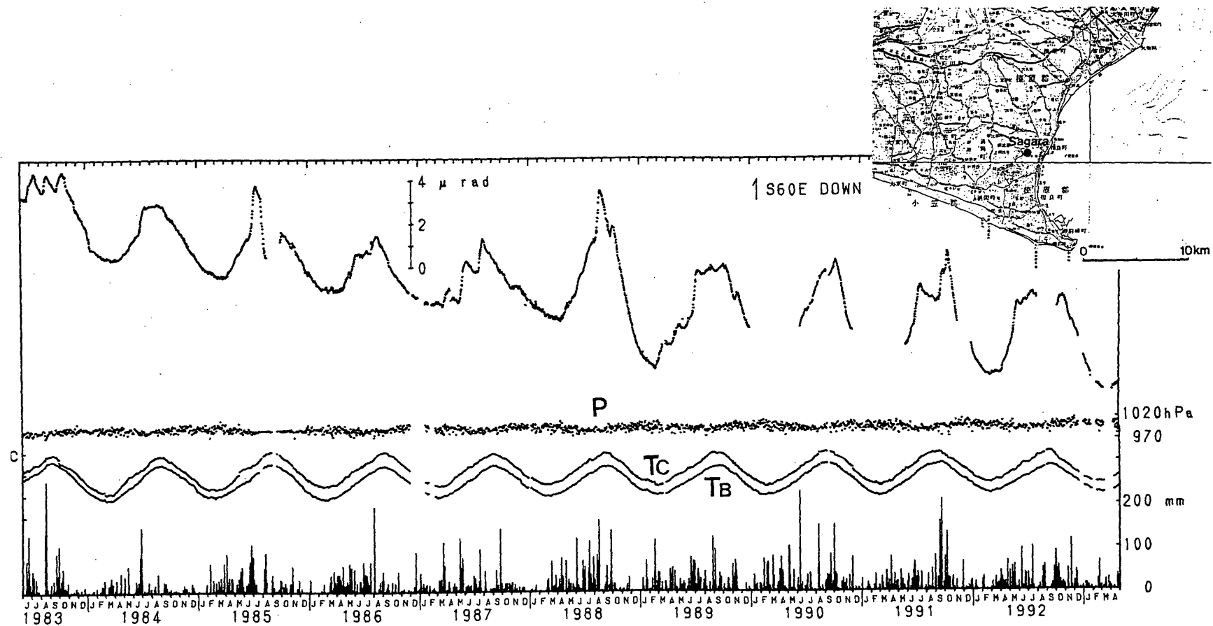
第1図 相良観測点での水管傾斜計による傾斜，気圧（P），傾斜計の中間点（T c ）と北西端（T b ）での温度の日平均値，および牧ノ原アメダスによる日雨量（1983年6月から1993年4月）
