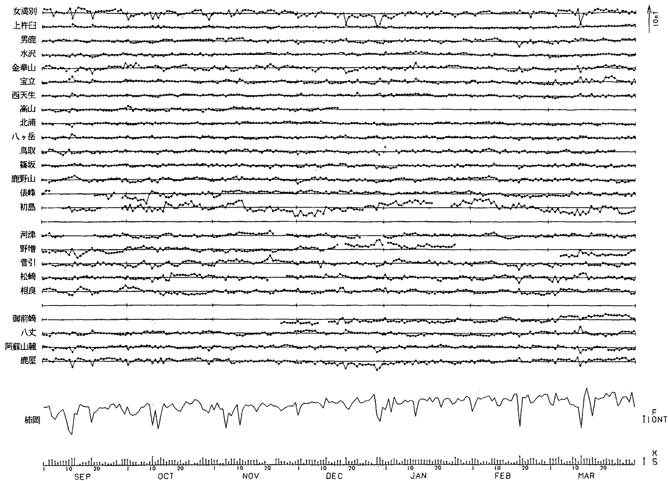
第3図 上段：拡張された主成分分析法により推定された，全磁力日平均夜間値の各観測点の局所的な変化。推定のための係数は1990年1～6月のデータに基づいて計算された。 下段：柿岡に於ける全磁力夜間値の日平均と夜間K指数 1992年9月～1993年3月
