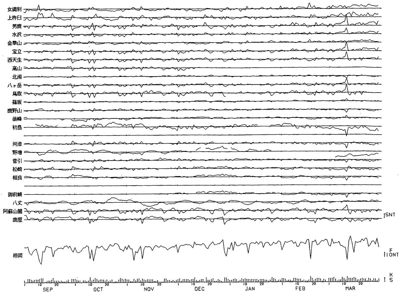
第2図 上段：柿岡に対する各観測点の全磁力夜間値の日平均値の重価差 下段：柿岡に於ける全磁力夜間値の日平均と夜間K指数。 1992年9月～1993年3月
