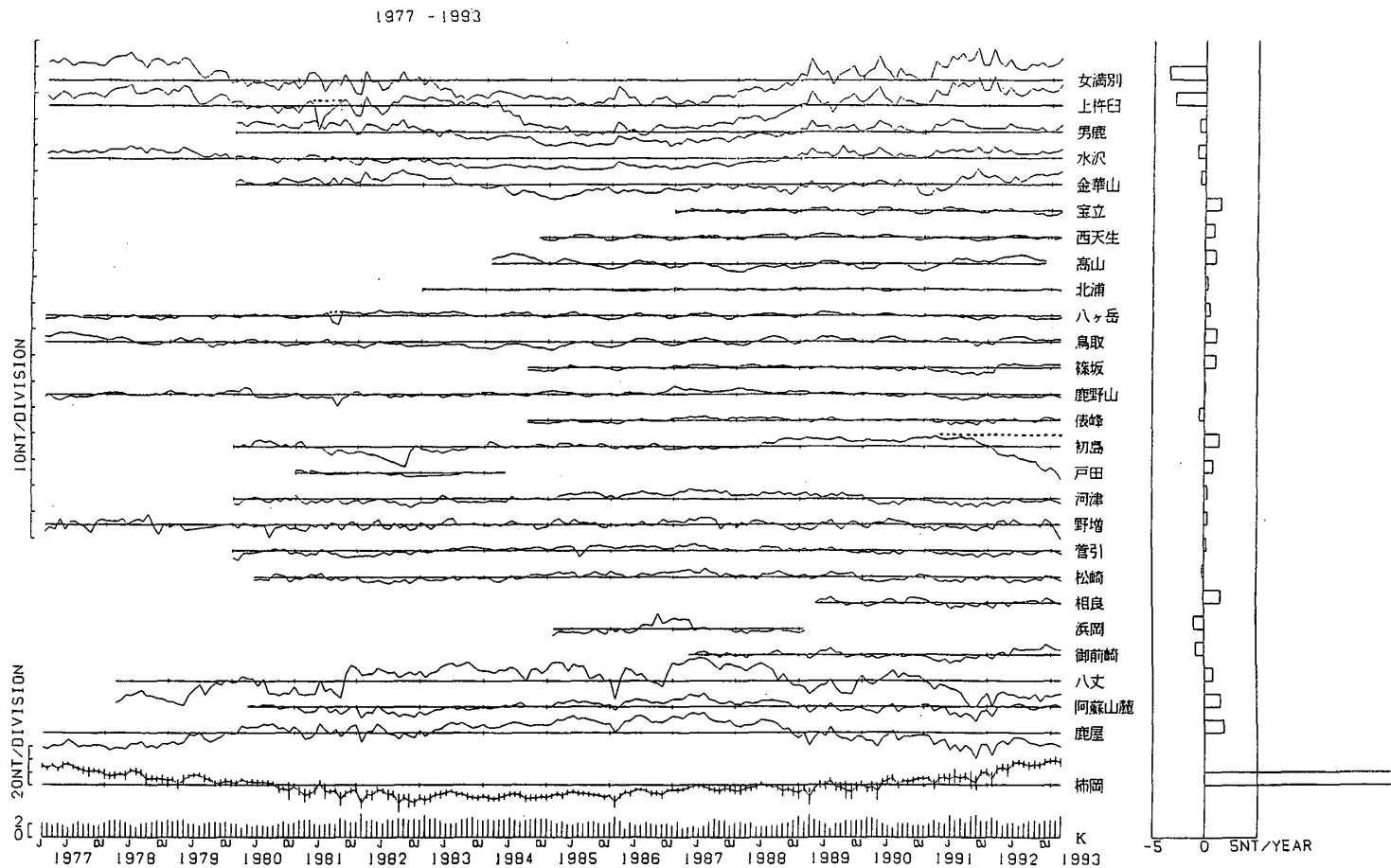
第4図 左：柿岡に対する各観測点の経年変化を除去した全磁力夜間値の単純差月平均値及び柿岡における全磁力夜間値と夜間K指数の月平均値
