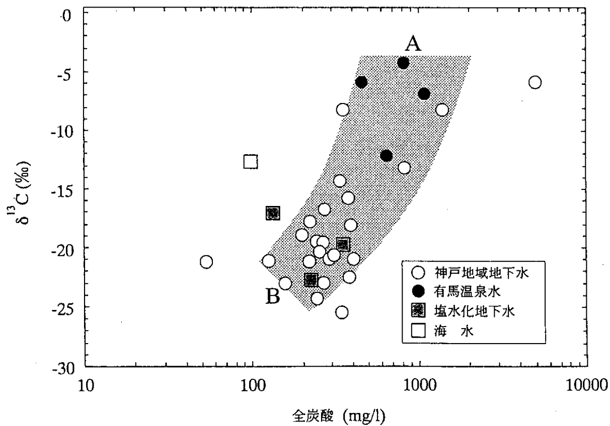
第4図 \delta^{13}\text{C} 値と全炭酸濃度との関係
