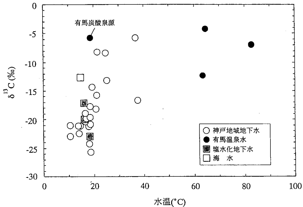
第3図 全炭酸の \delta^{13}\text{C} 値と水温との関係
