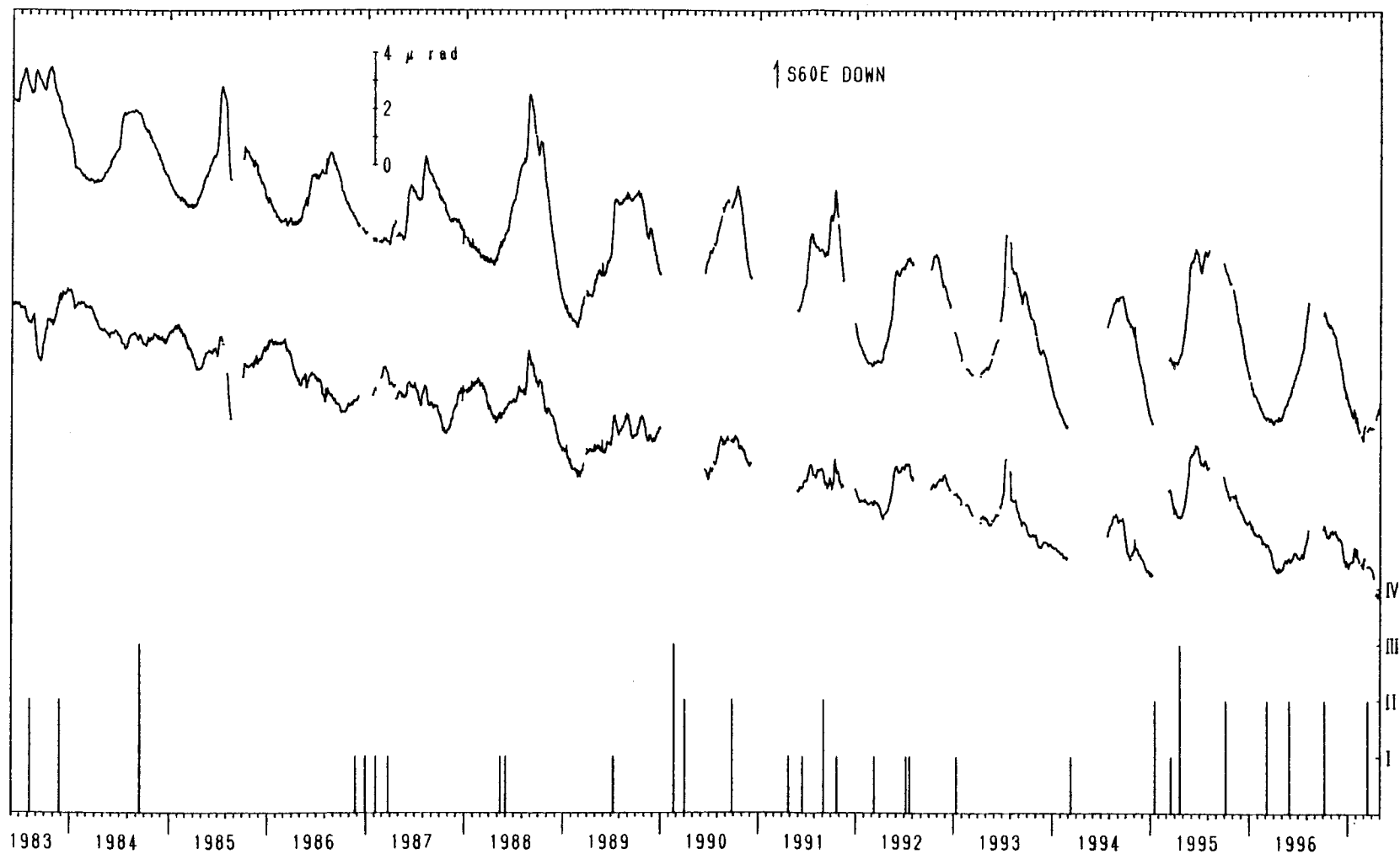
第2図 相良観測点の水管傾斜計の日平均値と、それから雨量と温度の影響を取り除いた結果。 縦線は御前崎における有感地震の震度。(1983年6月から1997年4月)
