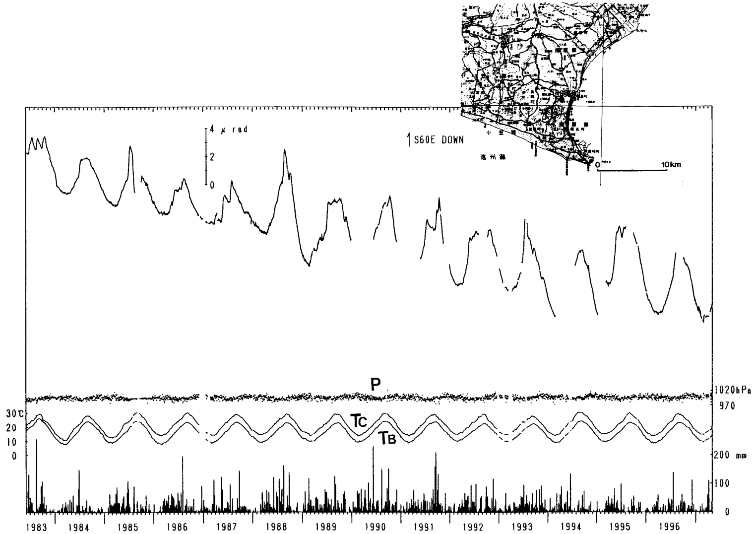
第 1 図 相良観測点での水管傾斜計による傾斜，気圧 (P)，傾斜計の中間点 (TC) と北西端 (TB) での温度の日平均値，および牧ノ原アメダスによる日雨量。(1983 年 6 月から 1997 年 4 月)
