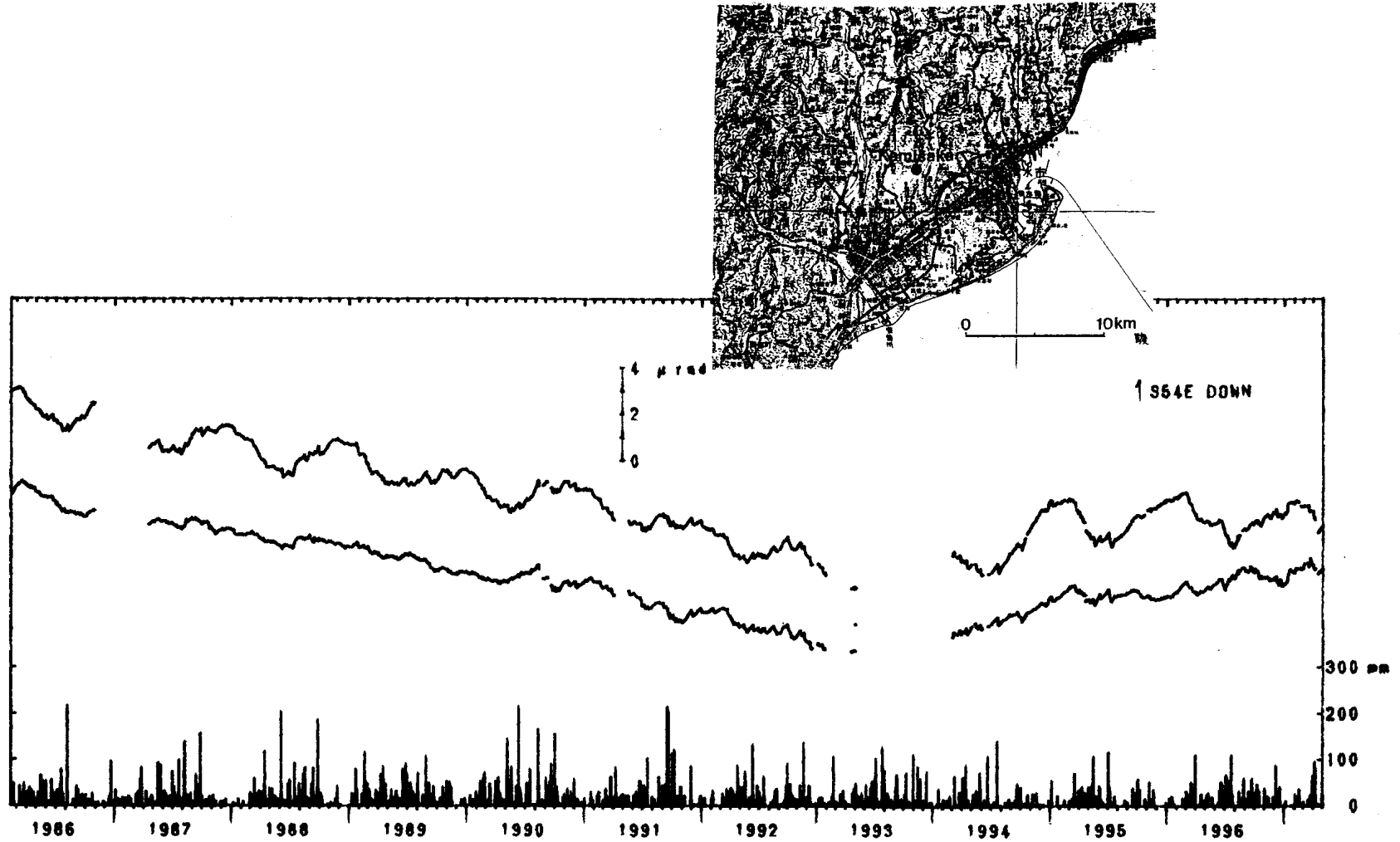
第3図 上坂観測点の水管傾斜計の日平均値と、それから年周変化と雨量の影響を取り除いた結果、 および静岡地方気象台での日雨量。(1986年2月から1997年4月)
