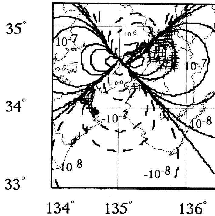
第1図 Hashimoto et al.(1996)のモデルから計算された，地表におけるコサイスミックな体積歪変化と観測井（×印）の分布。点線（負の値）が縮みで実線（正の値）が伸び。
