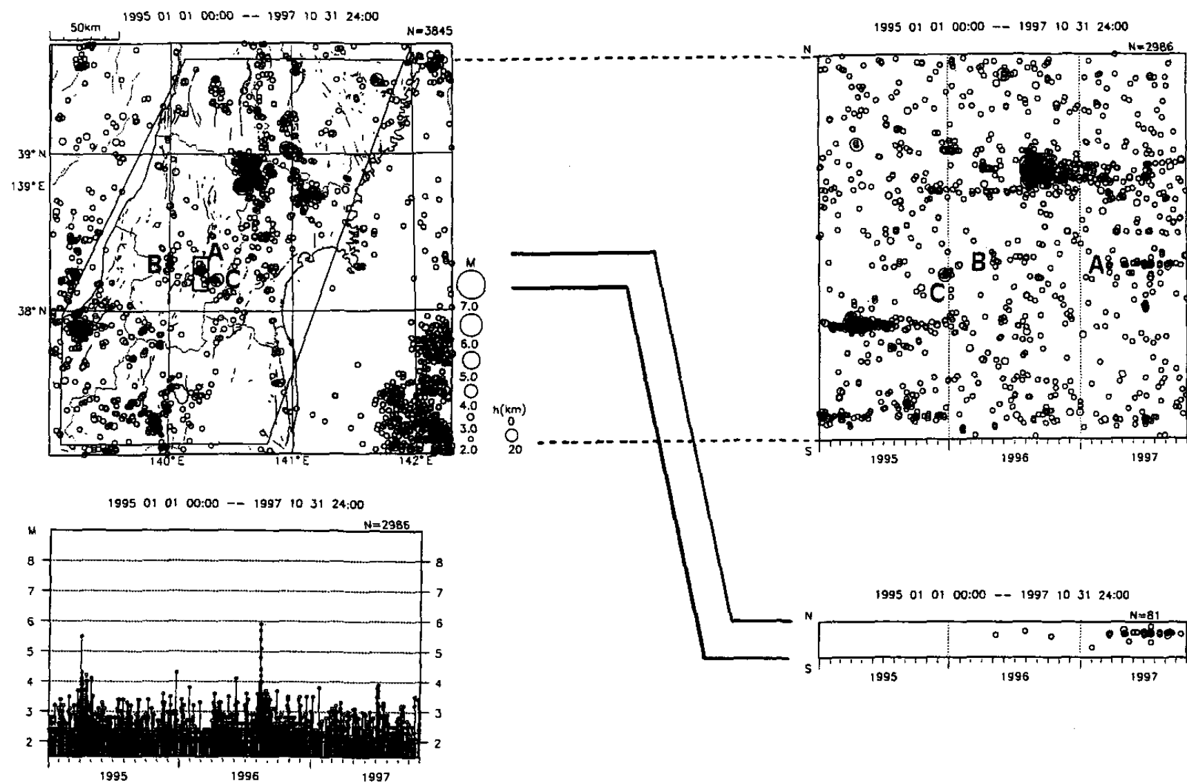
第1図 つづき(b)1995年1月1日~1997年10月31日 ( M 2.0 h 20km )
