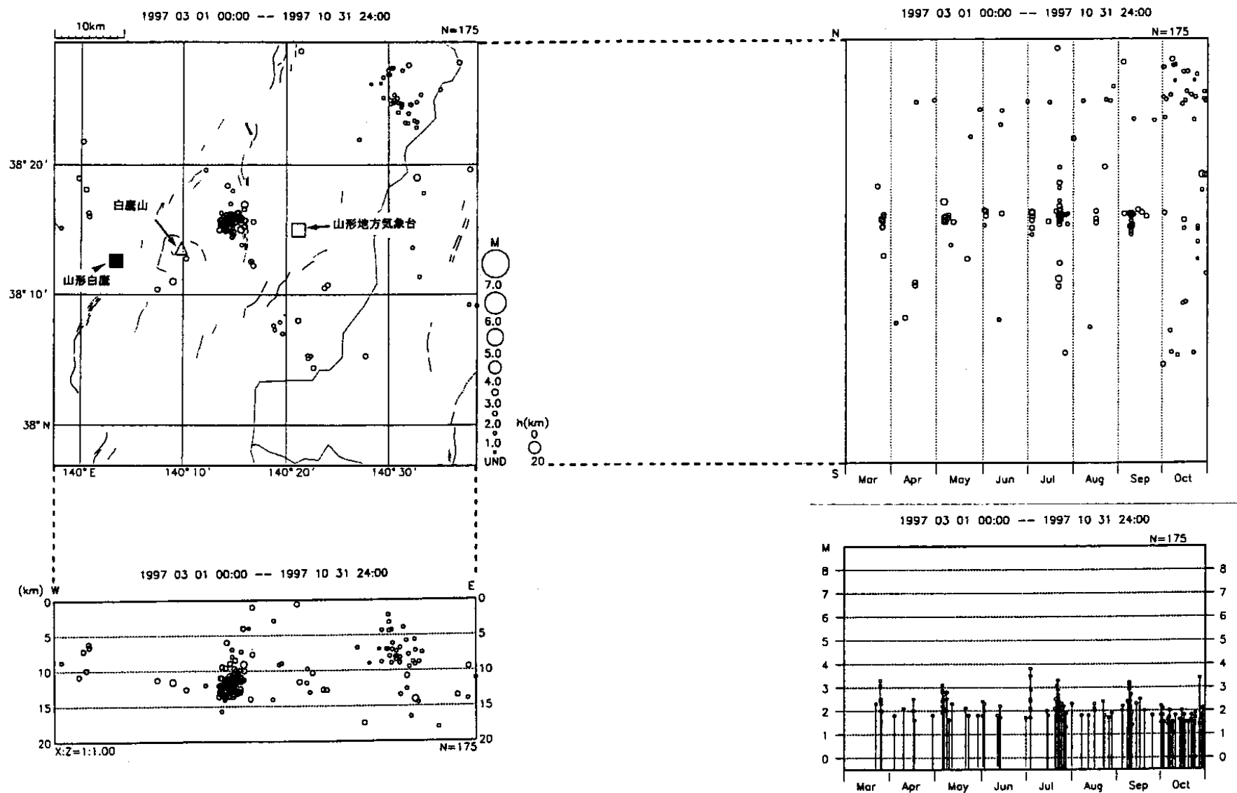
第1図 山形県村山地方の地震活動：(a)1997年3月1日～1997年10月31日 (h 20km)
