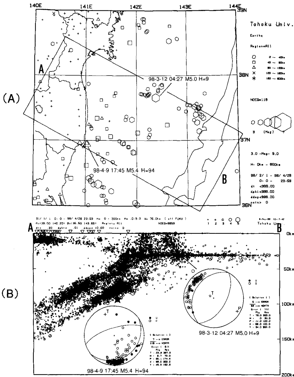
第1図 福島県沖の地震活動。(A) 1998年2月～4月28日に福島県沖に発生したM 3の地震の震央分布。図中の矩形領域A Bは第1図(B)の断面の位置を表す。(B) 1991年1月～1998年4月28日の期間に発生した地震の深さ分布。最近のM 5クラスの地震のメカニズム解を下半球等積投影で示す。
