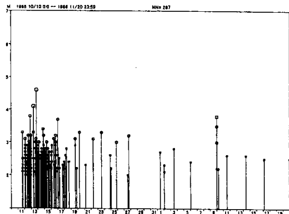
第3図 つづき (b)
