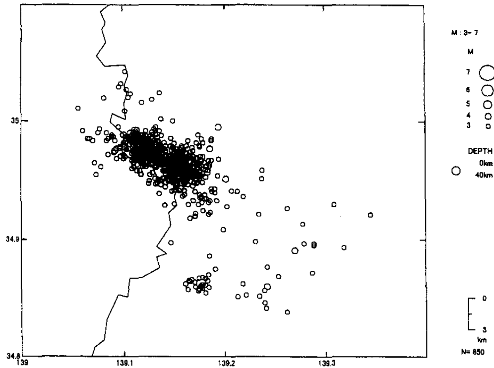
第2図 伊豆半島東方沖地震群の前期(上)と後期(下)の震央分布。
