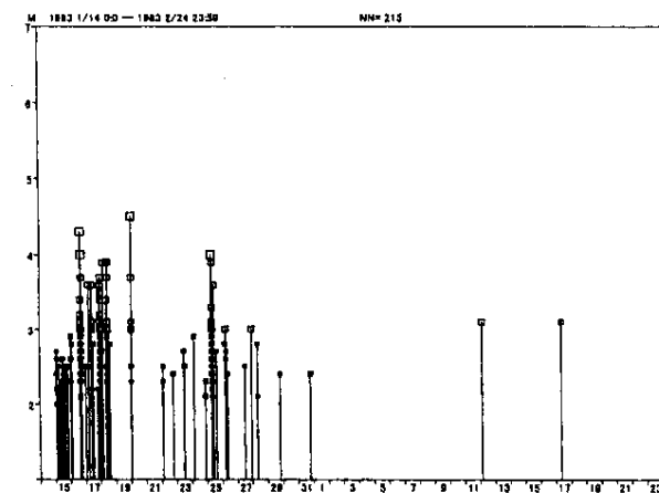
第3図 1978年以来の主な伊豆半島東方沖群発地震の震央分布図とM-Tグラフ (a)
