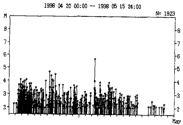
第3図 つづき (e)
