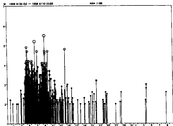
第3図 つづき (c) Fig.3 (Continued) (c)
