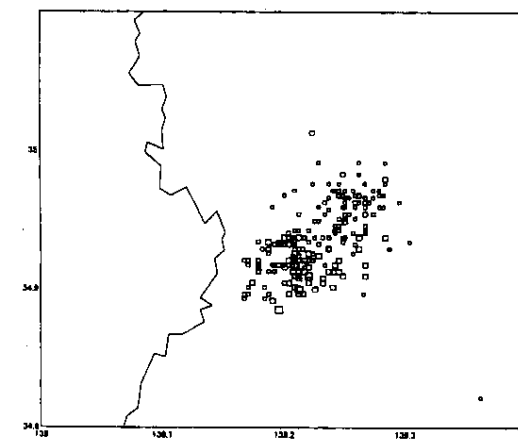
第3図 1978年以来の主な伊豆半島東方沖群発地震の震央分布図とM-Tグラフ (a)
