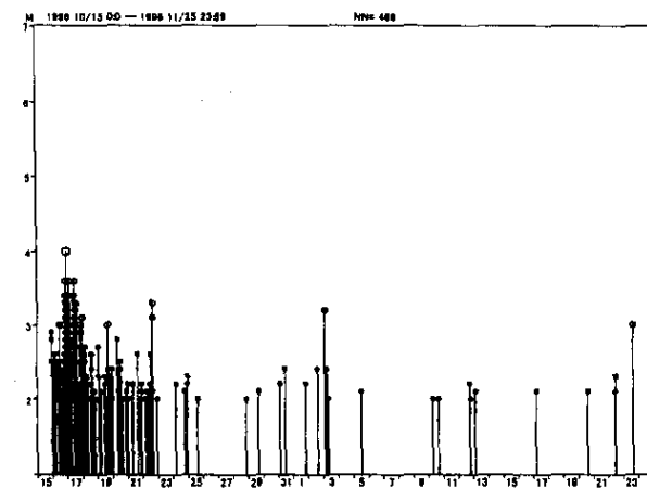
第3図 つづき (d) Fig.3 (Continued) (d)
