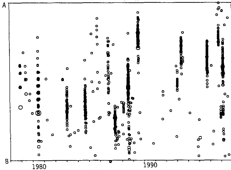
第 1 図 伊豆半島東方沖地震群 (1978 - 1997, M 3.0) の震央分布図 (上) と北西 - 南東方向 (AB) についての時空間分布図 (下)。データは気象庁。
