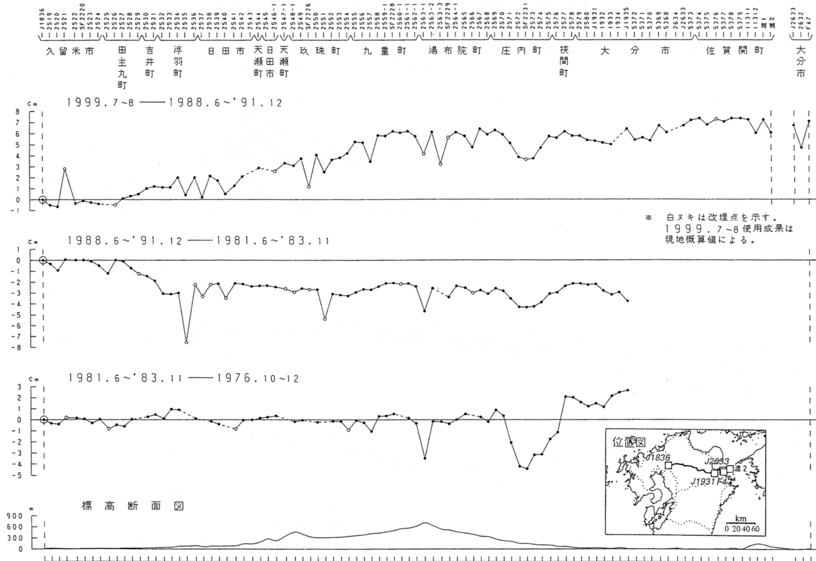
第1図 水準測量による九州北部地方の上下変動（久留米市～大分市）
