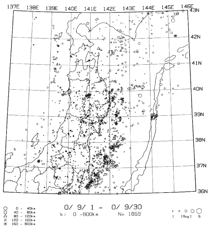
第9図 東北地方の微小地震の震央分布（2000年9月）
