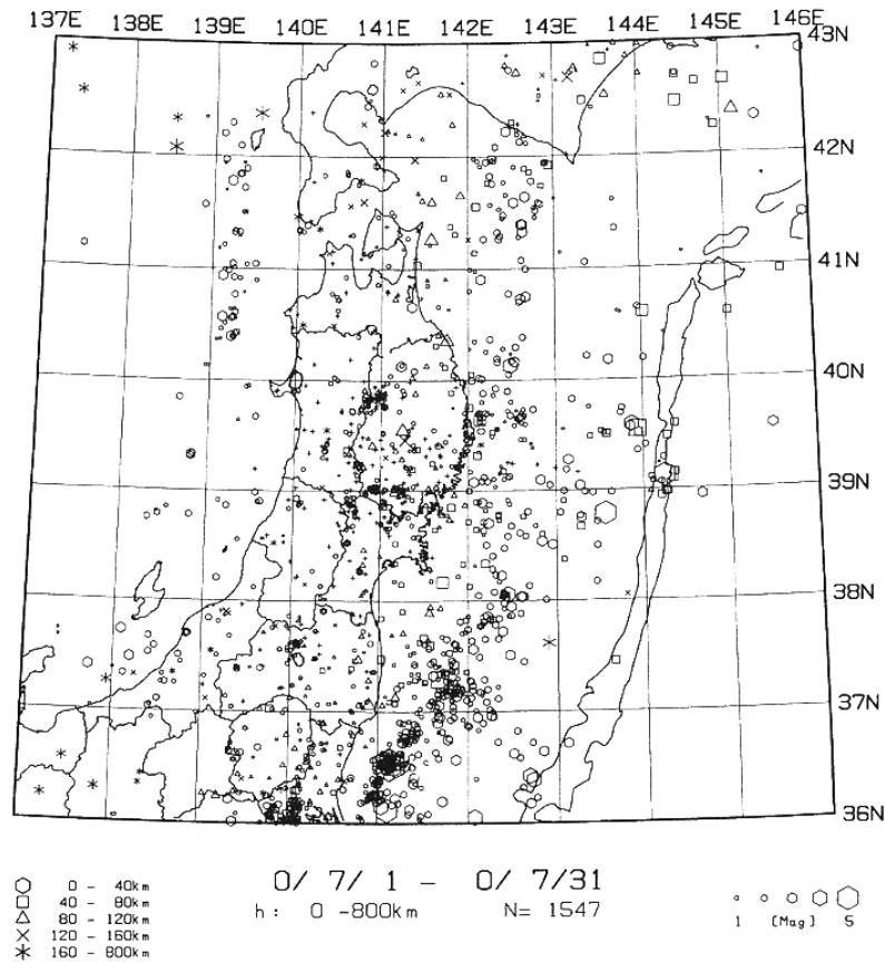
第7図 東北地方の微小地震の震央分布（2000年7月）
