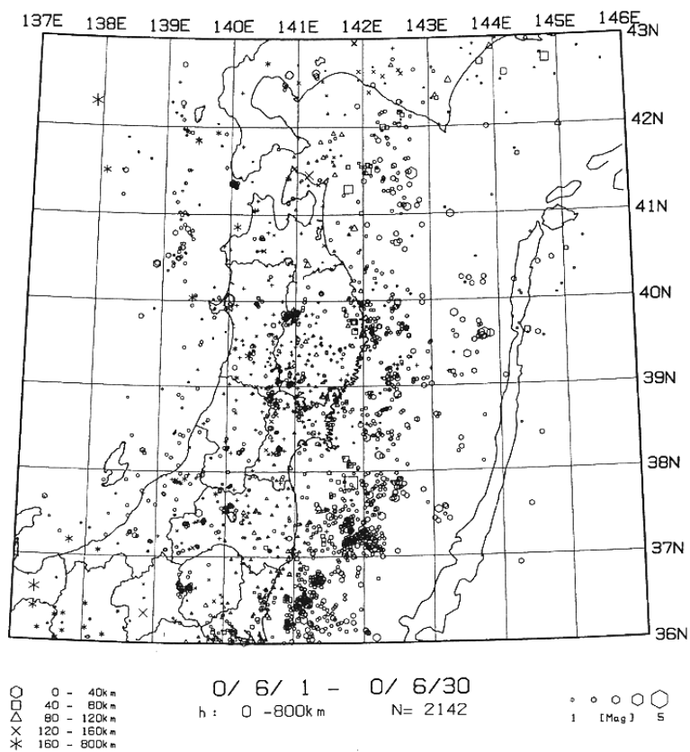
第6図 東北地方の微小地震の震央分布（2000年6月）
