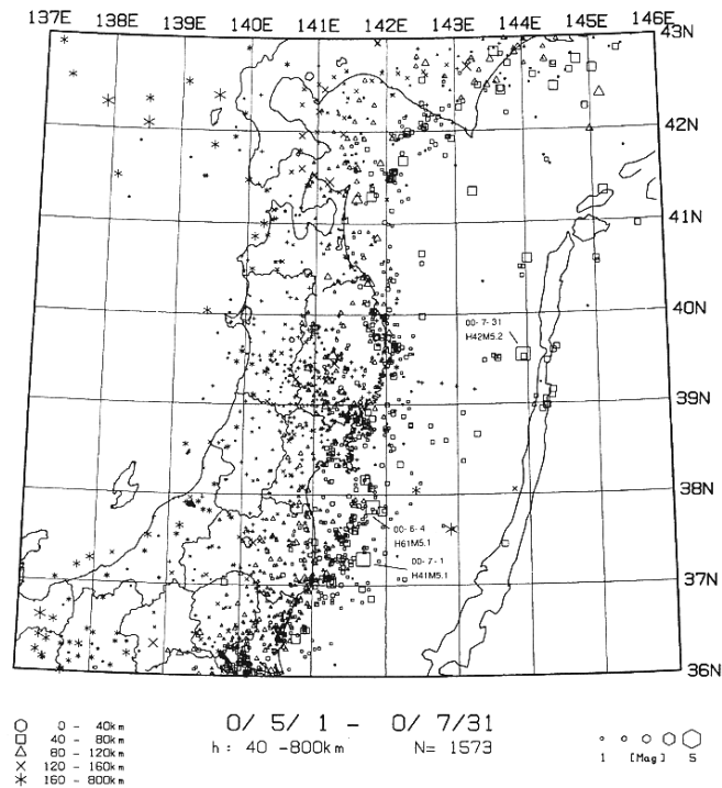
第3図 東北地方の h \geq 40 km の微小地震の震央分布 (2000年5月~7月)
