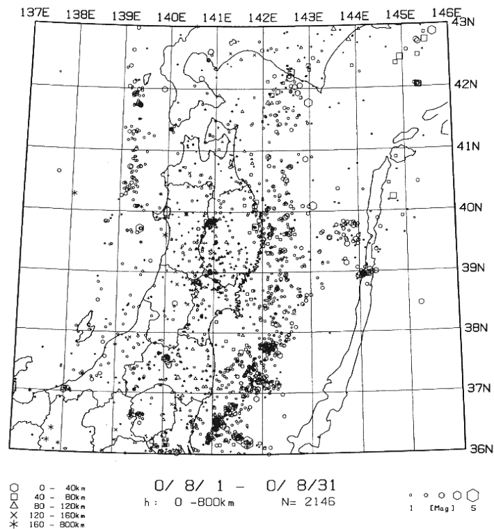
第8図 東北地方の微小地震の震央分布（2000年8月）
