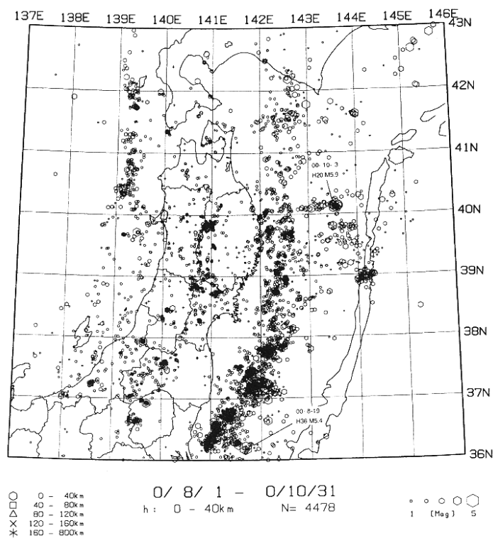
第2図 東北地方の浅発微小地震の震央分布 (2000年8月～0月)
