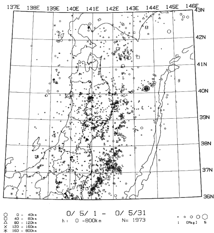
第5図 東北地方の微小地震の震央分布（2000年5月）
