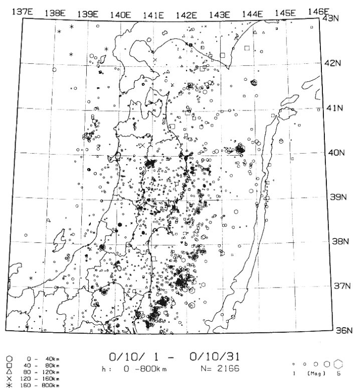
第10図 東北地方の微小地震の震央分布（2000年10月）
