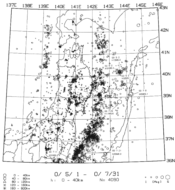
第1図 東北地方の浅発微小地震の震央分布 (2000年5月～7月)
