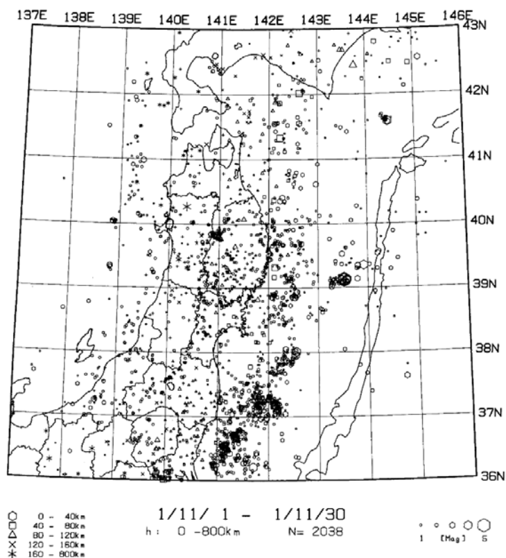
第 5 図 東北地方の微小地震の震央分布 (2001 年 11 月)
