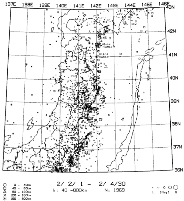
第4図 東北地方のh 40km の微小地震の震央分布 (2002年2月~4月)
