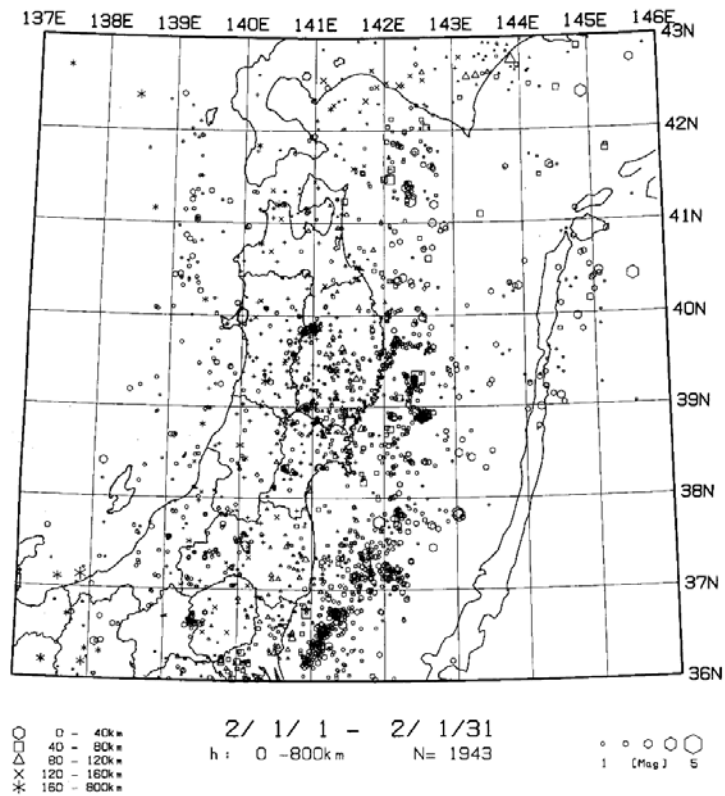
第7図 東北地方の微小地震の震央分布（2002年1月）
