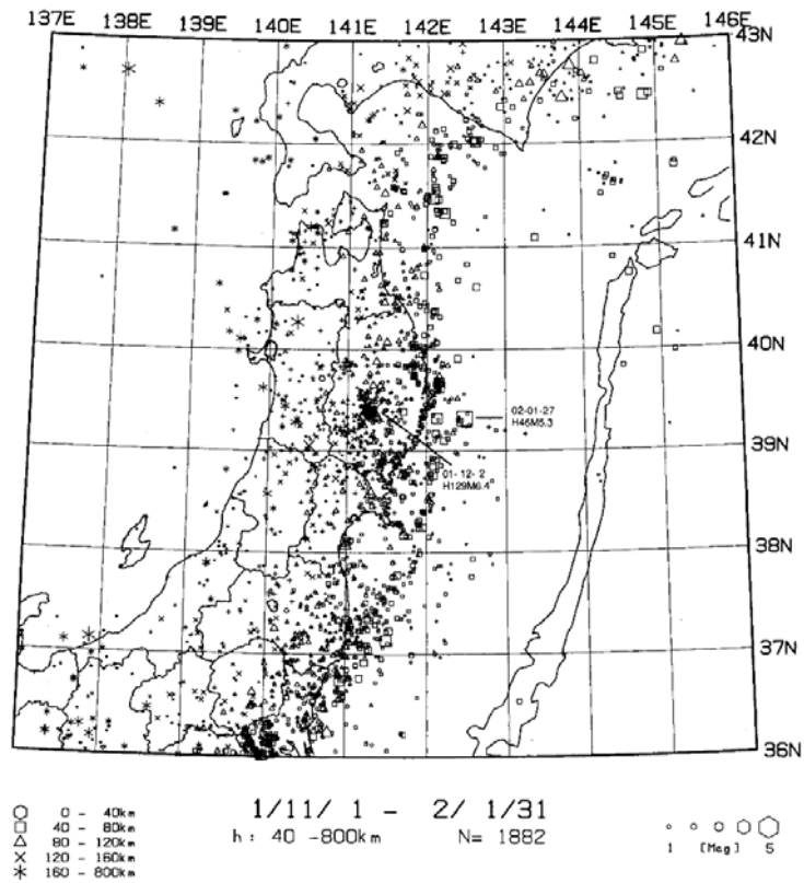
第3図 東北地方のh 40km の微小地震の震央分布 (2001年11月~2002年1月)
