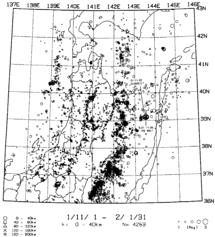
第1図 東北地方の浅発微小地震の震央分布 (2001年11月~2002年1月)
