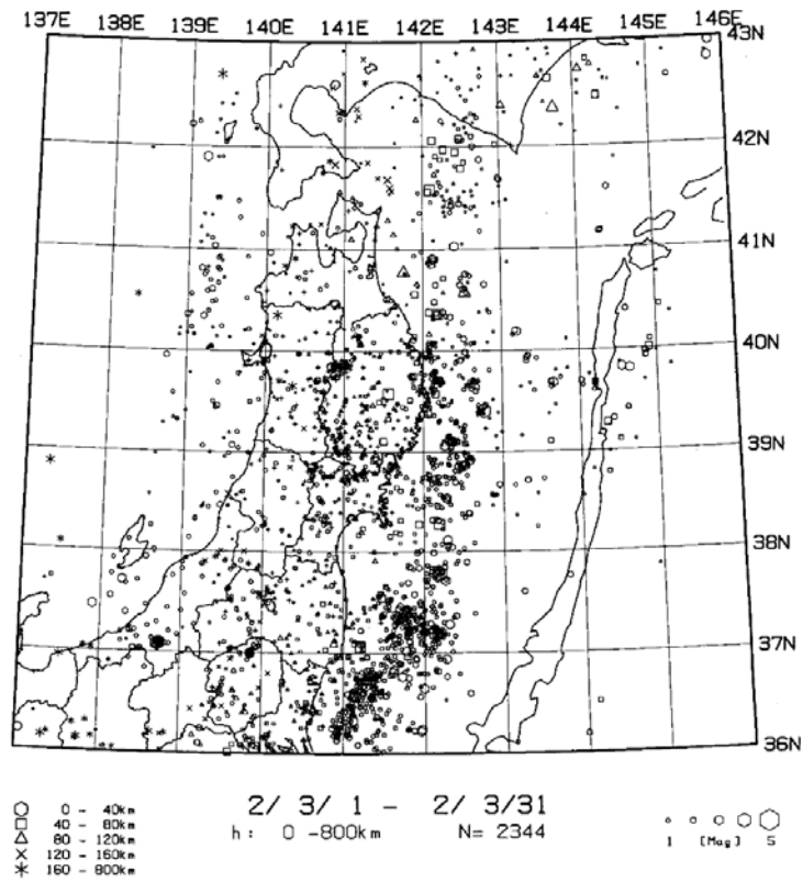
第 9 図 東北地方の微小地震の震央分布 (2002 年 3 月)
