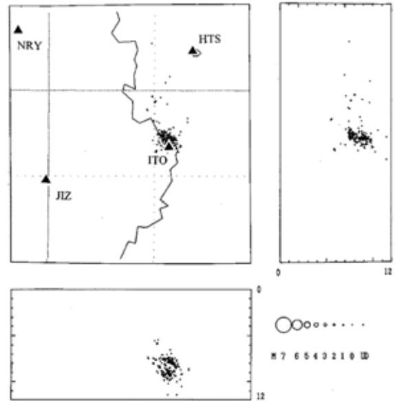
第 2 図 震源分布図 (2002 年 5 月 8 日 ~ 5 月 13 日) Fig.2 Hypocenter distribution for the period May 8 to 13, 2002.
