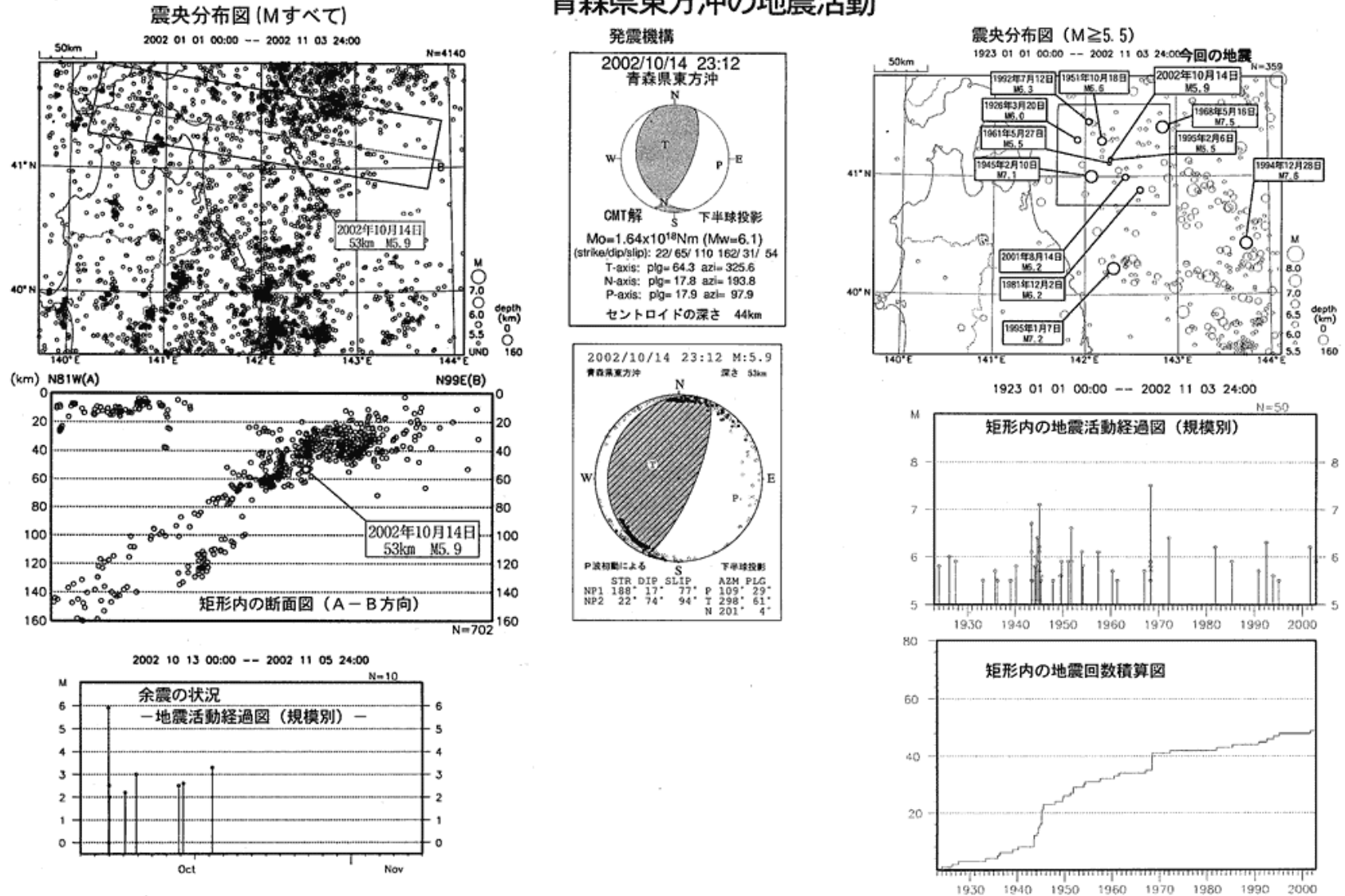
第1図 青森県東方沖の地震活動
