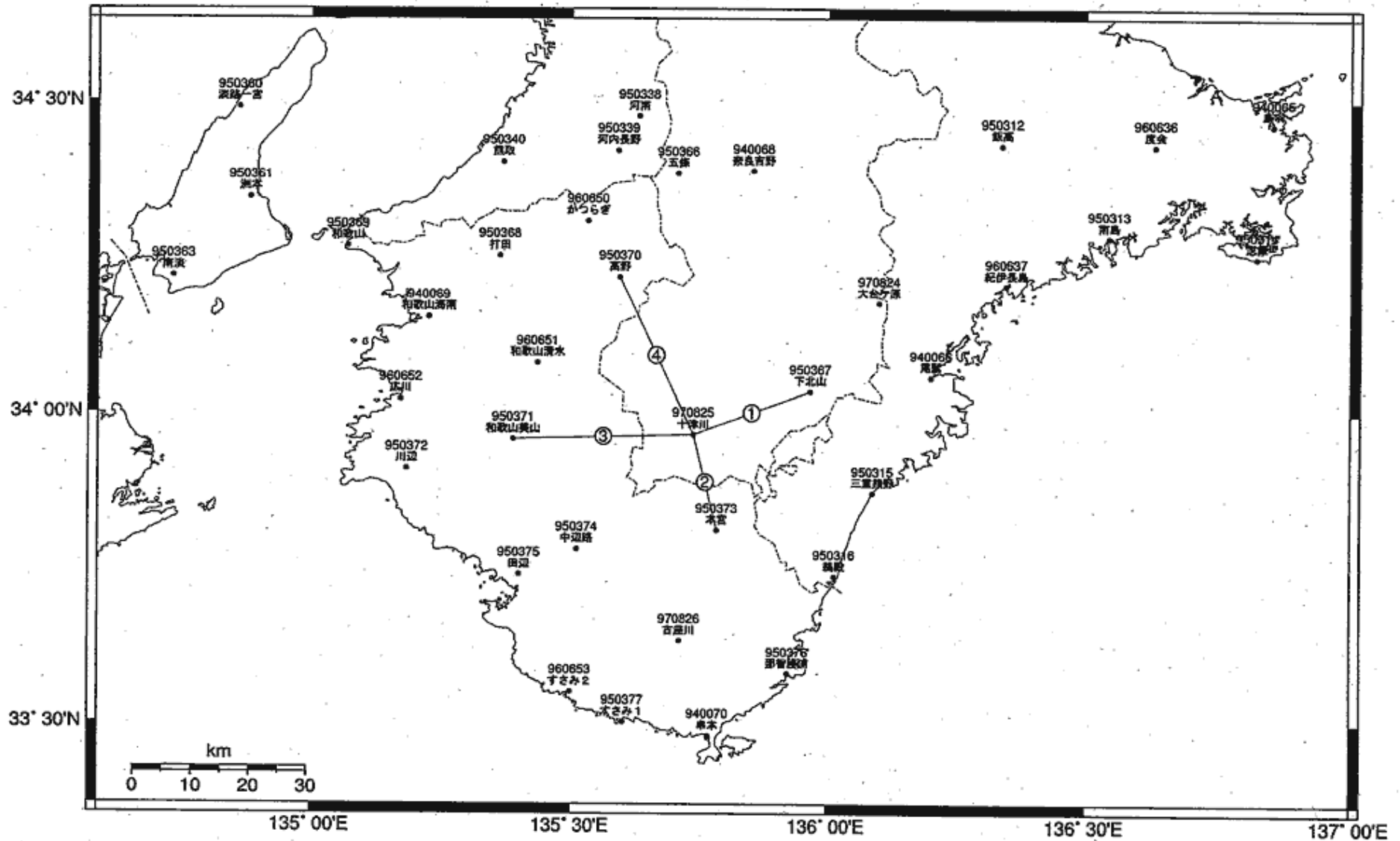
第1図 和歌山・奈良県境付近のGPS観測結果
