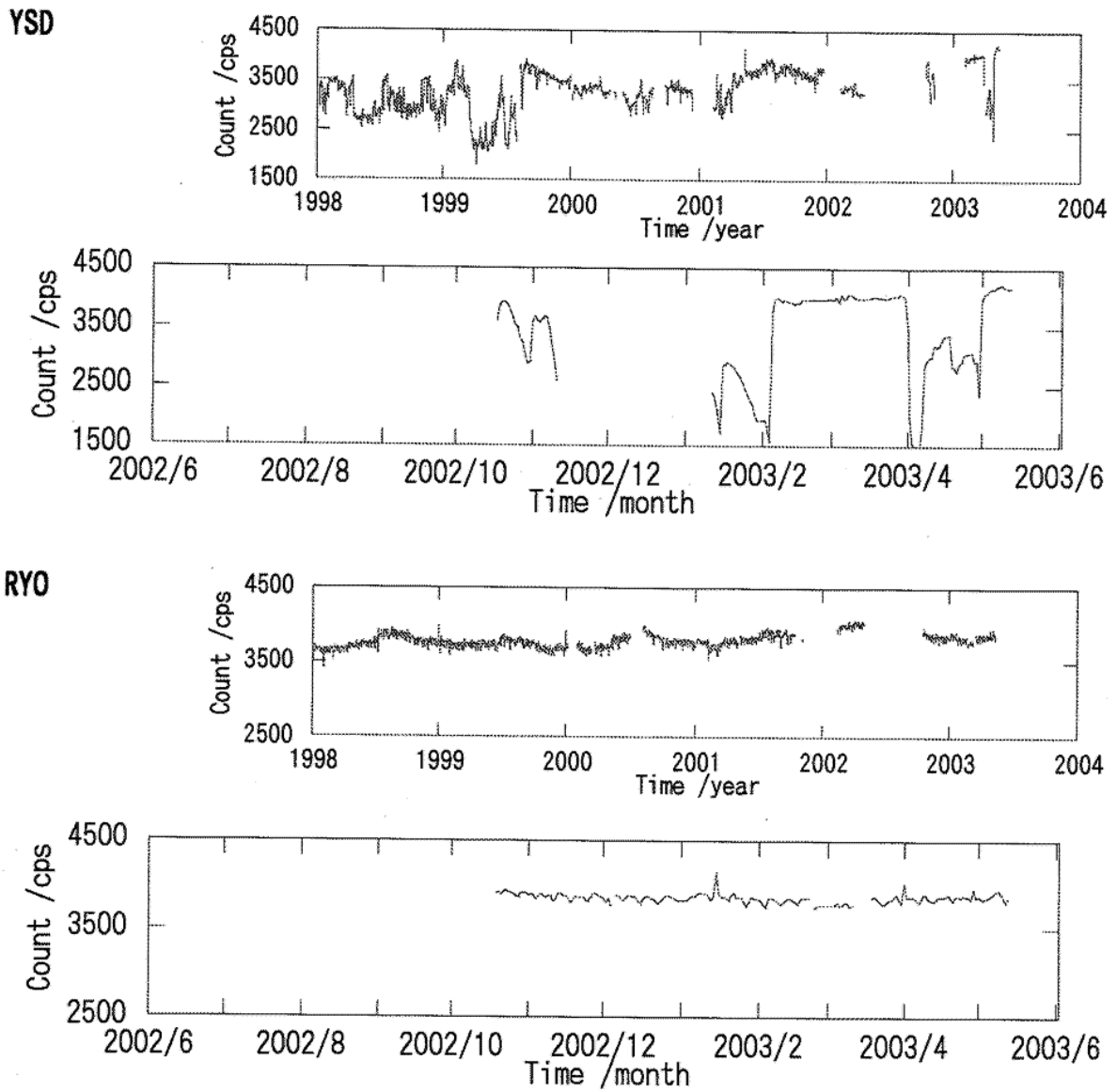
第 2 図 YSD、RYO における地下水のラドン濃度変化
