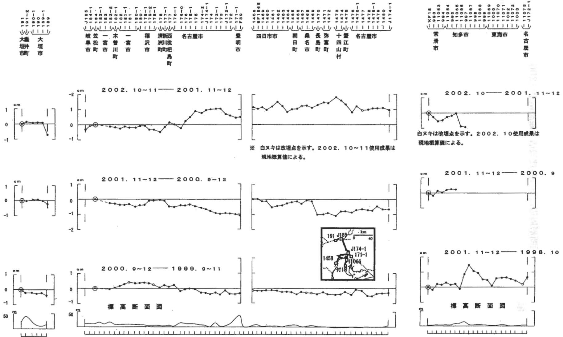
第1図 名古屋周辺の水準測量結果 Fig.1 Results of Precise Leveling around Nagoya city
