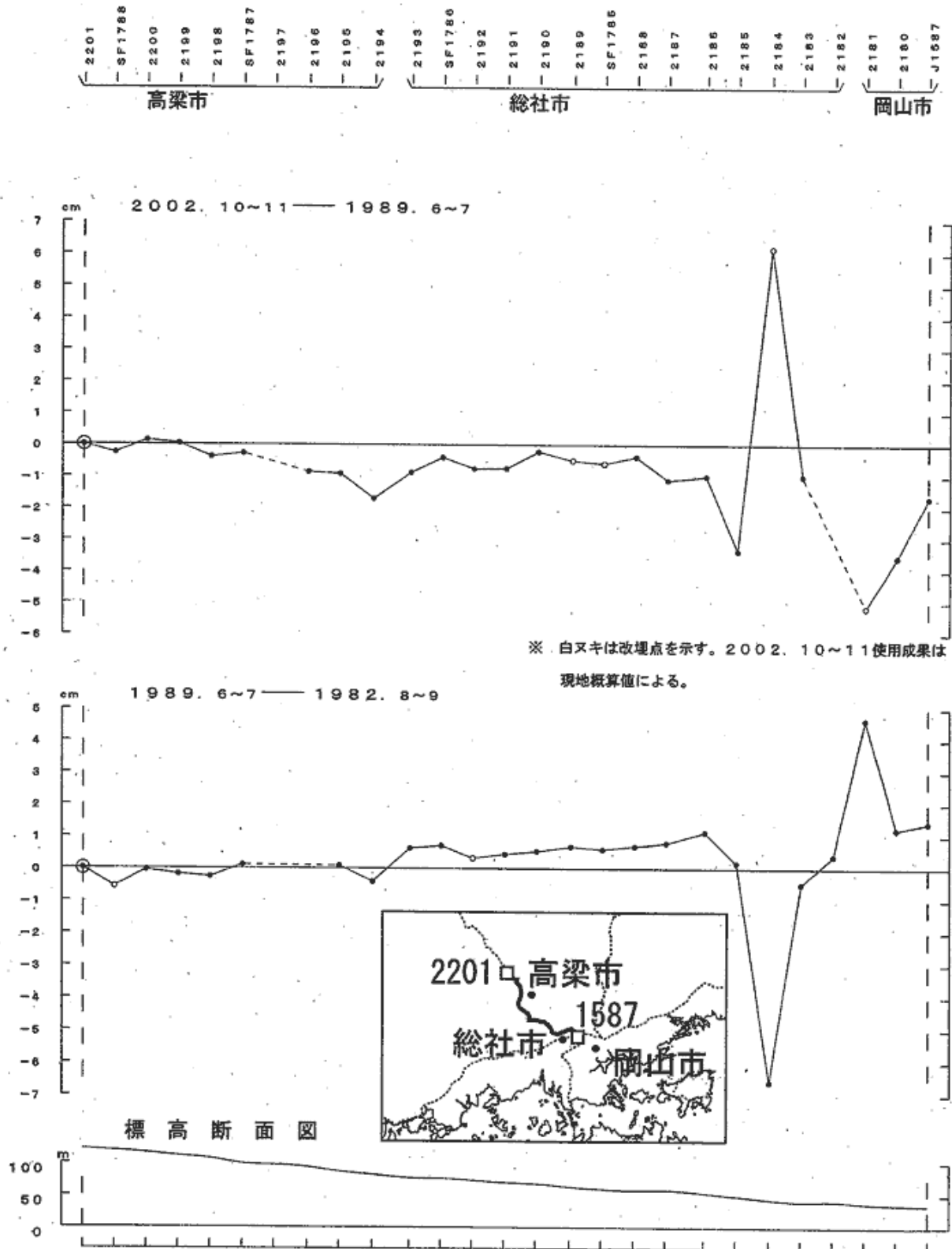
第1図 岡山県における水準測量結果
