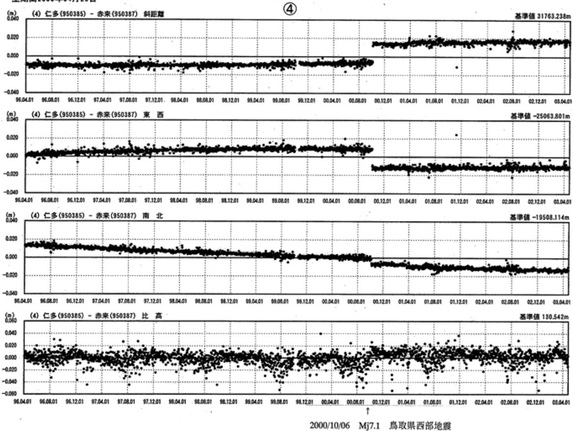
第4図 鳥根県東部のGPS連続観測結果
