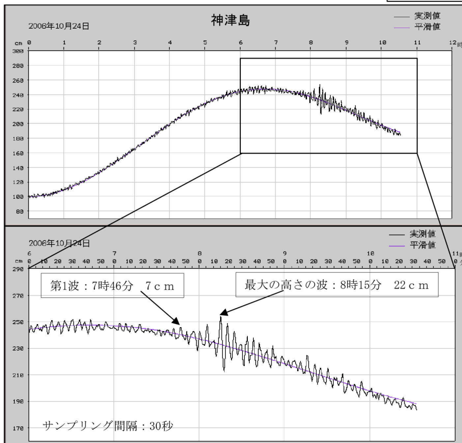
第1図 神津島験潮所の津波記録
