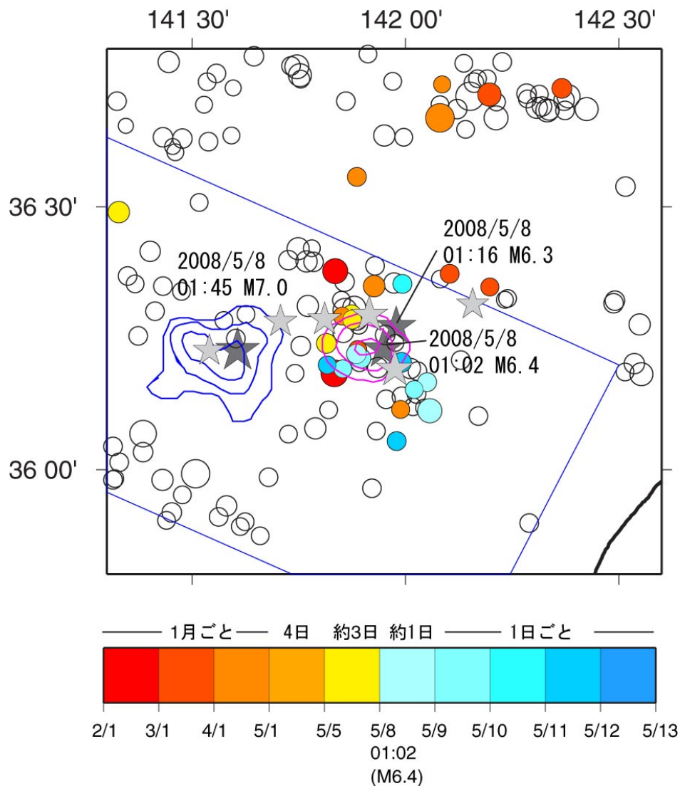
第2図 震源域周辺の小繰り返し地震グループの分布 (丸印). 2008年2月1日から5月12日までに地震が発生したグループは発生時に対応した色をつけて示す. グループの位置は, そのグループに属する地震の重心の位置であり, 上記の期間に2度同じグループで小繰り返し地震が発生したグループは存在しない. ピンク及び青のコンターは, 山中 (2008) による2008年5月8日 M6.4 および5月8日 M7.0 の地震のすべり量分布 (M6.4 は0.2m から0.1m 間隔, M7.0 は0.6m から0.3m 間隔) を示す. また, M5以上の地震の震央を薄い灰色, M6以上の地震の震央を濃い灰色の星印で示す. 青の線は図1と同様. M7.0 の地震のすべり域は, 小繰り返し地震があまり分布しない場所に位置する. M6.4 の地震前の小繰り返し地震 (暖色系) は, 地震時すべり域周辺~北の領域に分布する. 直前の期間には, すべり域に近いもの (黄色) が存在する. M6.4 およびM7.0 の地震後には, 主にM6.4地震のすべり域近傍やその海溝側で小繰り返し地震が発生している.
