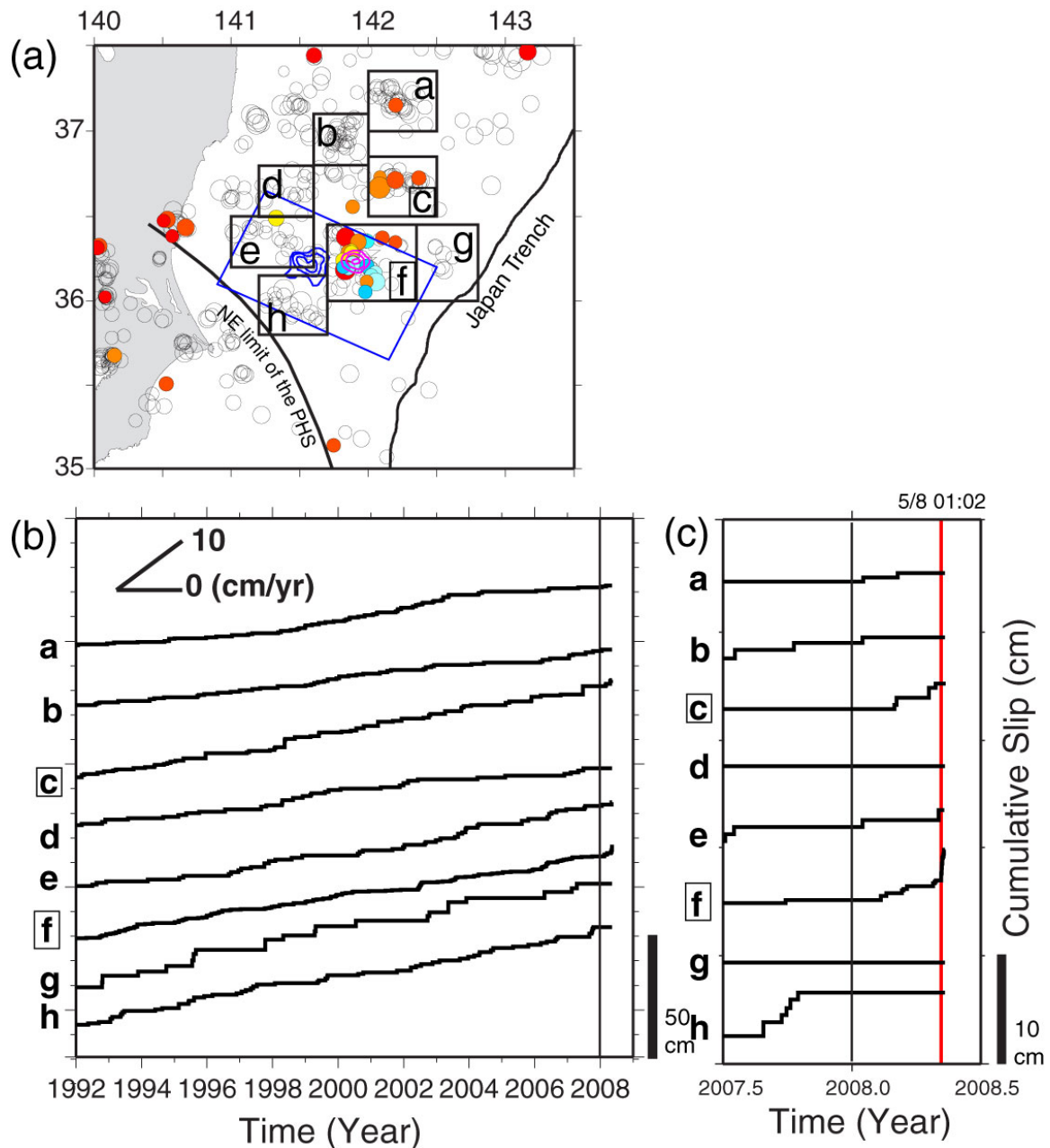
第3図 M7.0の地震の周囲の小繰り返し地震から推定した、プレート境界の準静的すべりの時間推移。(a) 推定に用いた小繰り返し地震グループの位置(丸印)。a-hの矩形で示した領域の平均のすべりを推定した。色がついている丸は、図2と同様に、2008年2月1日から5月12日までに地震が発生したグループでカラースケールも同様。コンター、青色矩形は図2、黒太線は図1と同様。(b) 1992-2008年5月12日の積算すべり。(c) 最近1年間の積算すべり。図b,cでは、黒の縦線で2008年1月1日、赤の縦線で2008年5月8日のM6.4の地震の発生時を示した。データの最後(線の右端)は、2008年5月13日。
