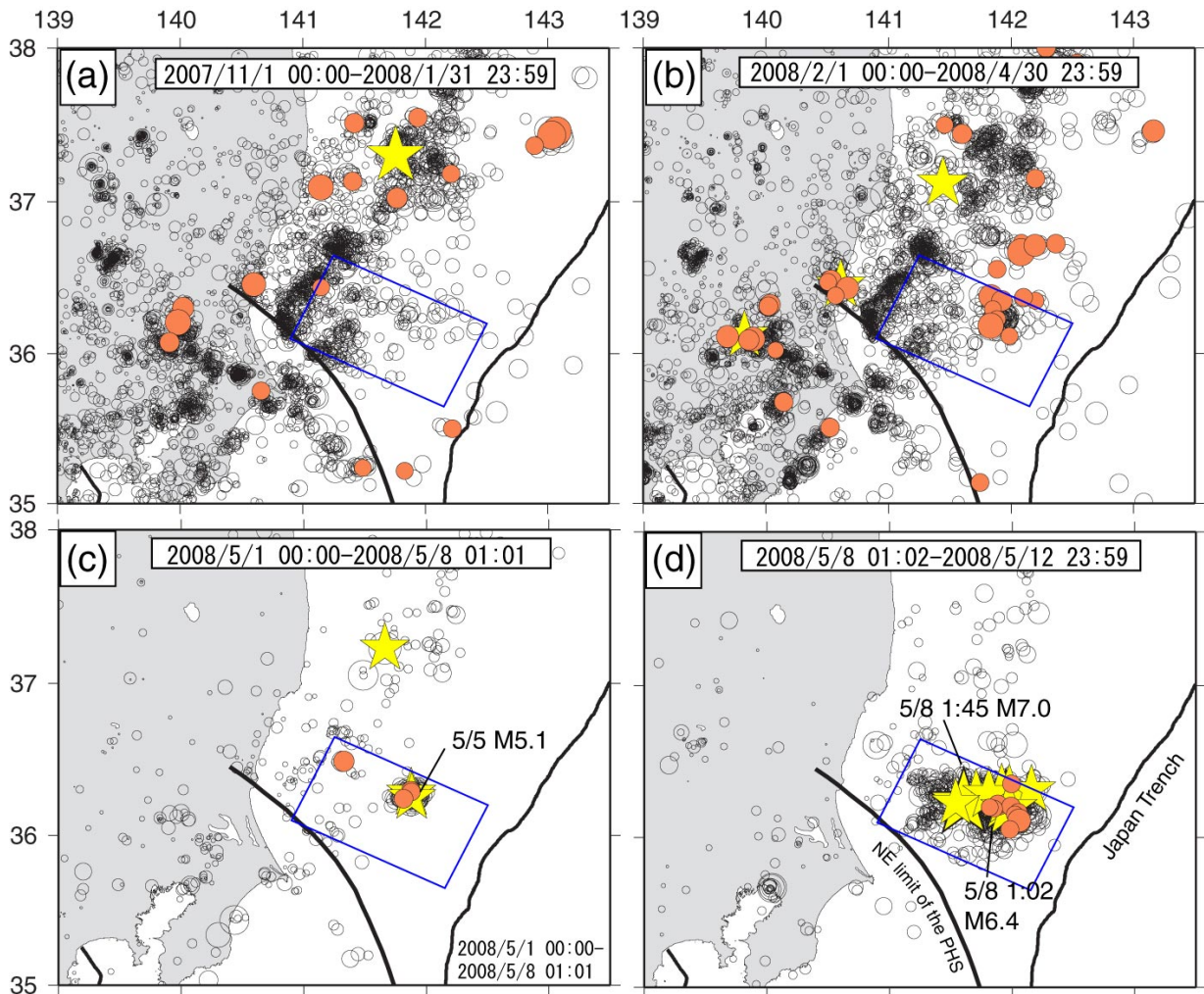
第1図 福島・茨城県沖の地震活動。気象庁による震源を丸印，そのうちの小繰り返し地震を橙色丸，M5以上の地震を星印で示す。期間は，(a)2007年11月1日-2008年1月31日，(b)2008年2月1日-4月30日 (c)2008年5月1日-5月8日1時1分(M6.4の地震前まで)，(d)2008年5月8日1時2分-5月12日。太線はフィリピン海プレートの北東端(内田・他，2007)，青色矩形はM7.0の地震の余震活動が活発な領域を示す。2008年2月頃から，M6.4の地震の周辺やその北方で小繰り返し地震の活動が活発であった。なお，小繰り返し地震の，同定は，内田・他(2007)と同様の波形の相関を用いた方法を用い，1992年以降の地震を解析した。解析には，東北大学の観測点のほか東京大学の観測点を用いた。
