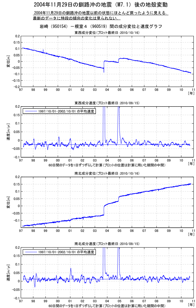
第7図 北海道太平洋岸の GEONET 観測点における地殻変動速度の変化(根室4観測点・時系列)
