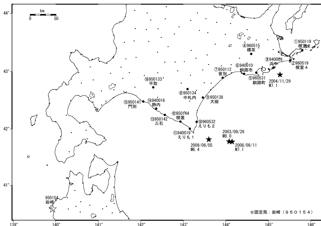
基線図
