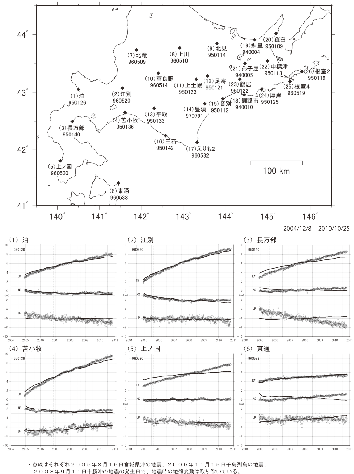
第 11 図 2004 年釧路沖の地震以降における観測された非定常地殻変動とモデルによる計算値とを比較した時系列
