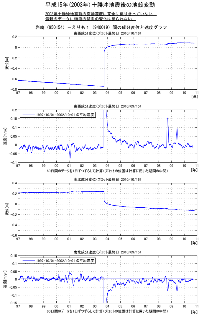
第6図 北海道太平洋岸の GEONET 観測点における地殻変動速度の変化(えりも1観測点・時系列)
