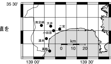
第2図 2010年5月-2010年7月の観測結果. Fig. 2 Observational results from May 2010 to July 2010.
