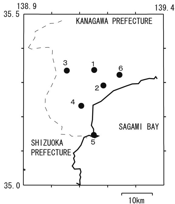
第1図 神奈川県温泉地学研究所の地下水観測点の分布(●). 1:大井, 2:小田原, 3:南足柄, 4:湯本, 5:真鶴, 6:二宮の各観測点. Fig. 1 Distribution of groundwater observation stations of Hot Springs Research Institute of Kanagawa Prefecture (●). 1:Ooi, 2:Odawara, 3:Minami-ashigara, 4:Yumoto, 5:Manazuru, 6:Ninomiya.
