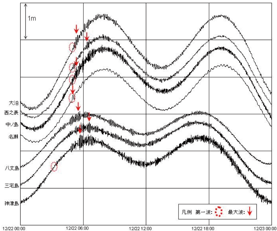
第2図 海上保安庁所管の験潮所で得られた津波記録(2010/12/22) Fig.2 Tsunami records at the tidal stations of Japan Coast Guard(December 22,2010).
