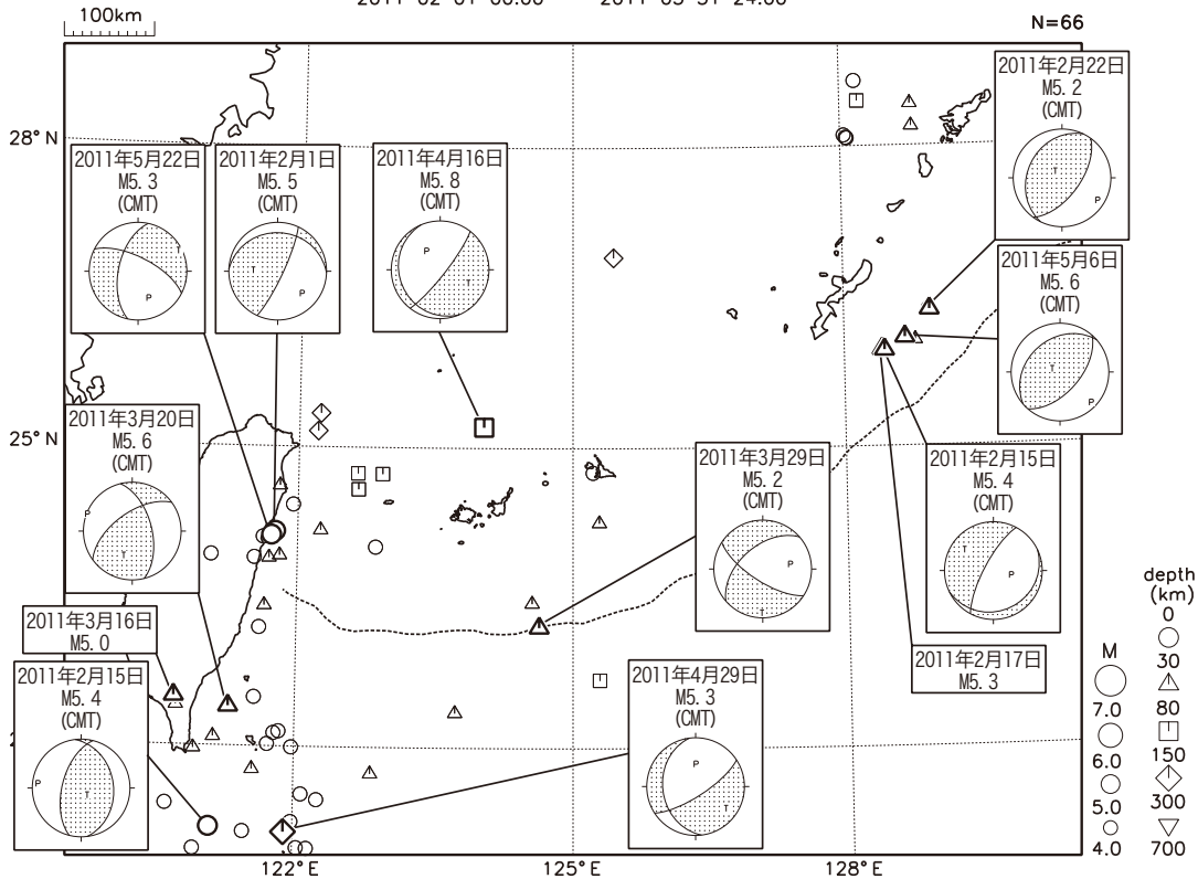
第1図(b) つづき(2011年2月~5月、M \geq 4.0、深さ \leq 700km) Fig.1(b) Continued (February - May 2011, M \geq 4.0, depth \leq 700km).
