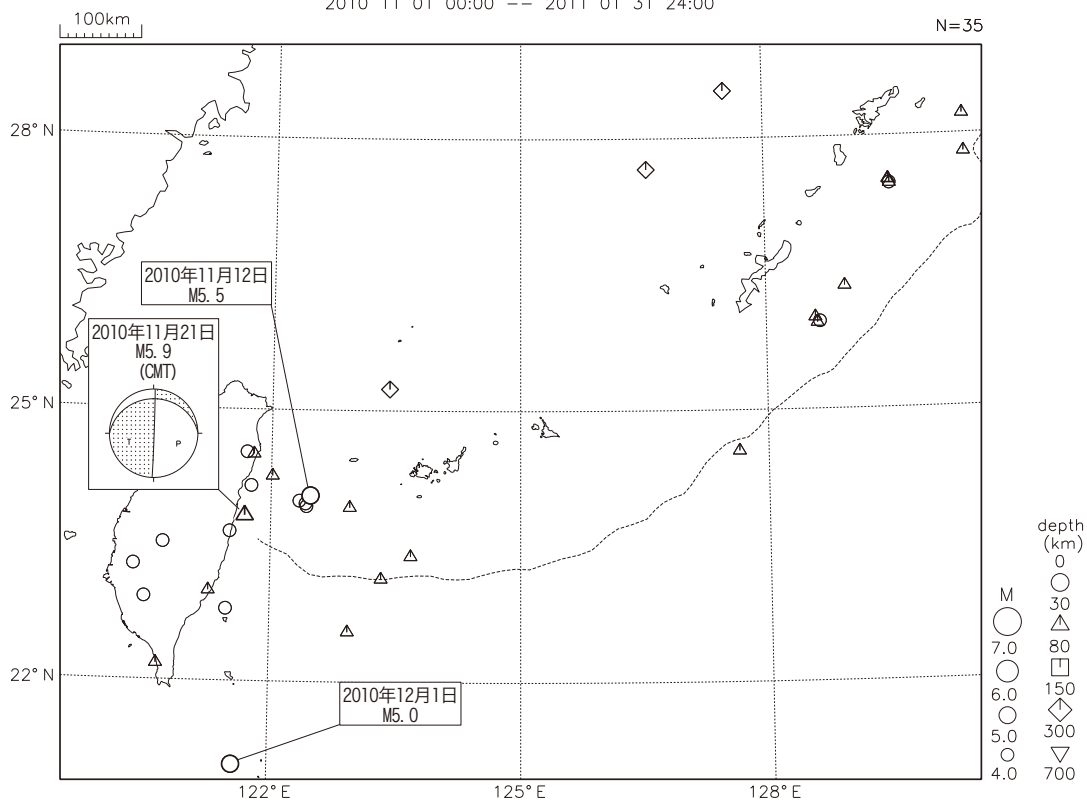
第1図(a) 沖縄地方とその周辺の地震活動(2010年11月~2011年1月、M \geq 4.0、深さ \leq 700km) Fig.1(a) Seismic activity around the Okinawa district (November 2010- January 2011, M \geq 4.0, depth \leq 700km).
