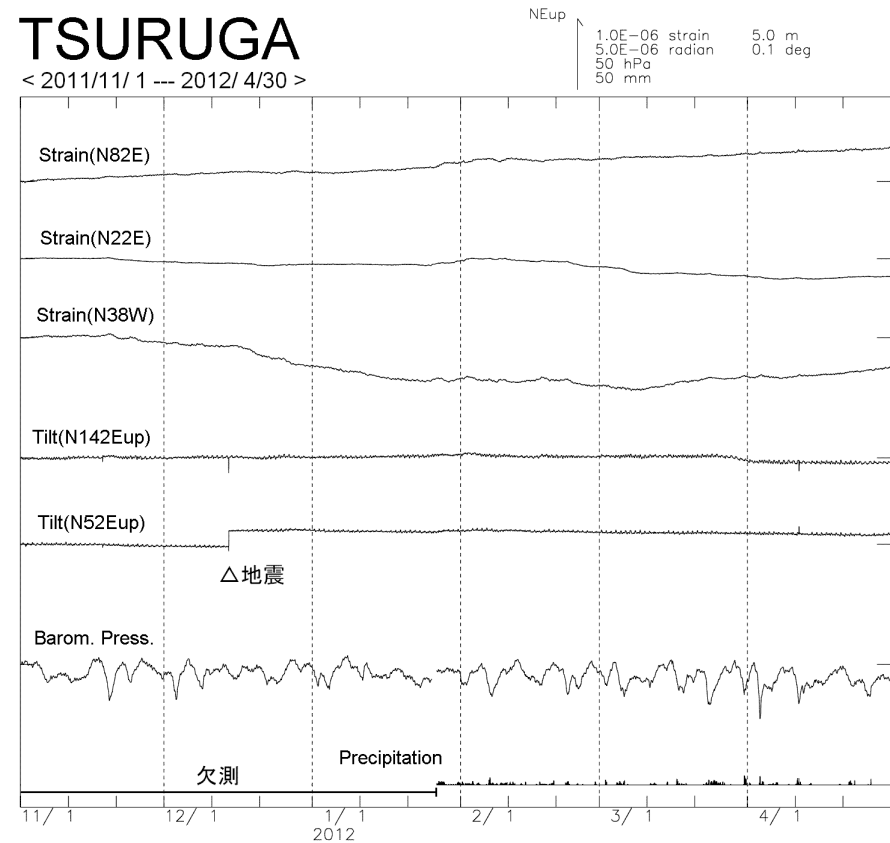
第3図 敦賀観測点における(上) 2009年5月～2012年4月, (下) 2011年11月～2012年4月のひずみ・傾斜変化(時間値). 2009年11月, 2010年6月, 7月, 8月のひずみ変化は温度計故障のため. 傾斜 N52Eup 成分に 2009年7月頃から見られる変化の原因は不明. ひずみ N38W 成分には毎年冬に縮み変化が見られるが, 変化の原因は不明.
