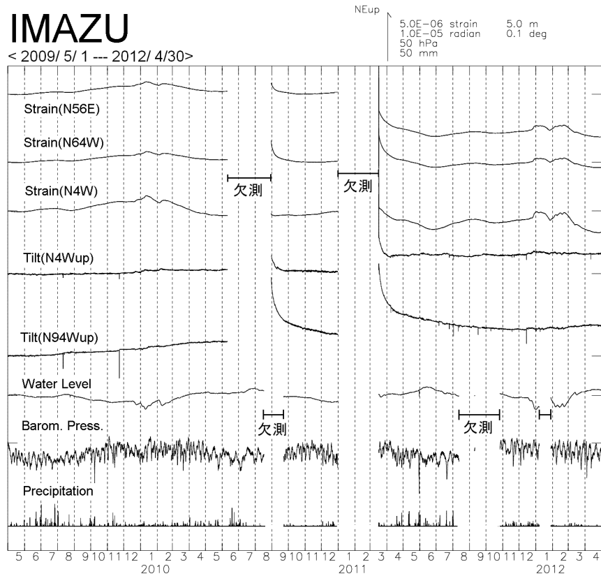
第 2 図 今津観測点における(上) 2009 年 5 月～2012 年 4 月, (下)2011 年 11 月～2012 年 4 月のひずみ・傾斜変化 (時間値). 毎年 1 月から 3 月のひずみ・水位変化は, 観測点付近の融雪のための地下水汲み上げに伴うもの.
