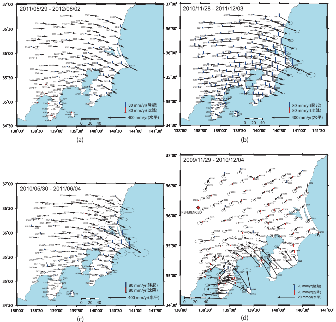
第2図 関東地方の2009年11月29日から2011年6月2日までの、半年ずつずらせた1年間ずつの地殻変位速度。水平成分の誤差楕円は1 \sigma (68 %) の誤差を示す。(d)では基準点の I G S 白田観測点に対する変位速度。
