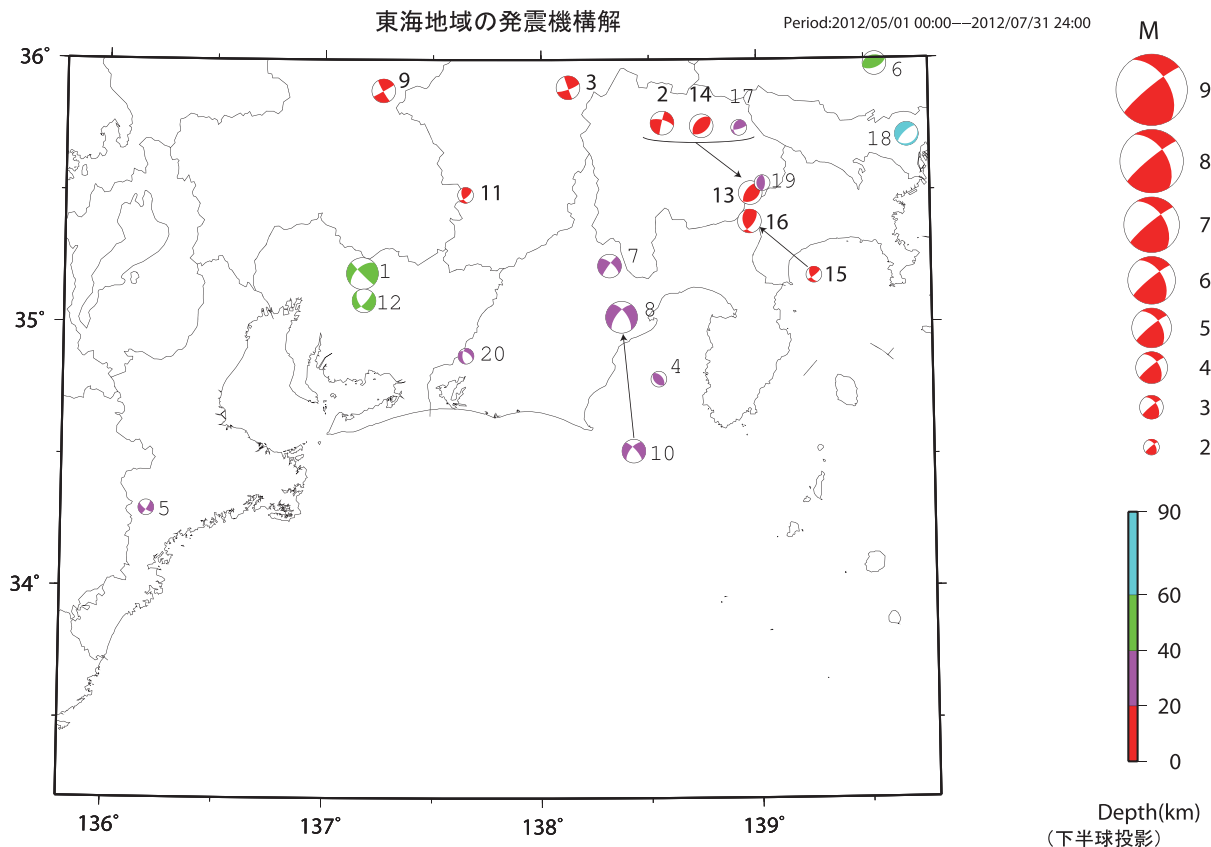
第2図(a) 東海で発生した主な地震の発震機構解 (2012年5月～7月)
