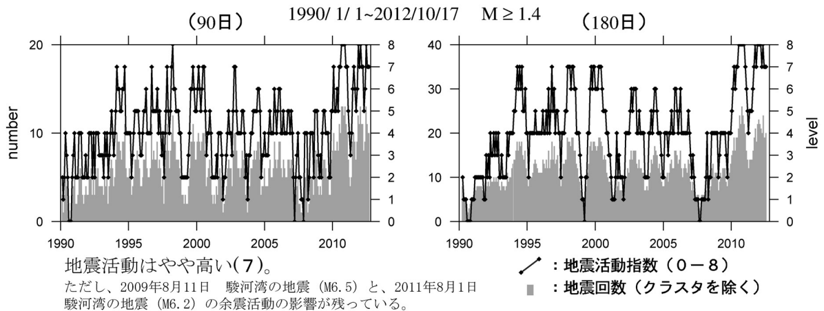
第13図 浜名湖及び駿河湾の地震活動指数の推移（浜名湖は1995年以降、駿河湾は1990年以降、第318回地震防災対策強化地域判定会気象庁資料 11) より抜粋）[指数算出の単位期間は90日と180日であり、全て30日ごとに指数をプロットしている。]
