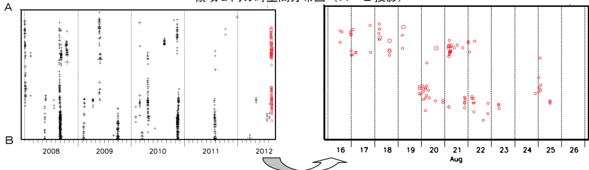
第4図(a) 2012年8月に長野県南部から愛知県で観測された深部低周波地震活動と短期的スロースリップ
