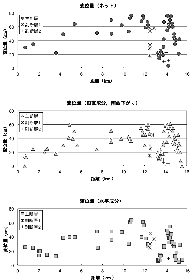
第1図 湯ノ岳・藤原断層に沿った地震断層の変位量分布. 北西端を距離0 km とする. Fig. 2 Slip distribution on the surface ruptures along the Yunodake and Fujiwara faults.
