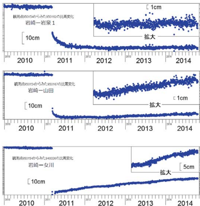
第3図 東北地方の比高変化（2010年1月から2014年10月）. Fig. 3 Time series of height difference in Tohoku district.
