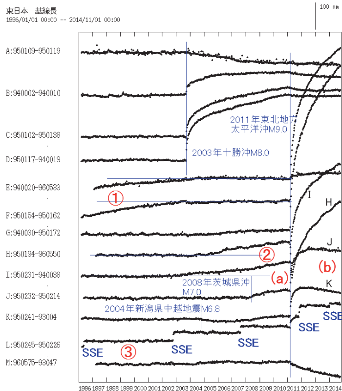
第2図(a) 基線長変化 (1996年から2014年10月) .
