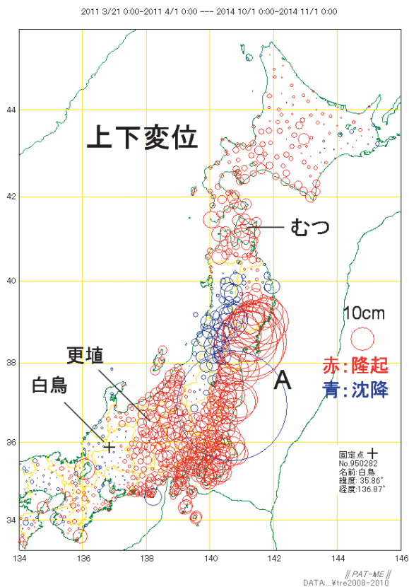
第4図 東北地方太平洋沖地震後（2011/3/21-31から2014/10）の非定常上下変位. Fig. 4 Unsteady vertical displacements after the 2011 off the Pacific coast of Tohoku Earthquake.
