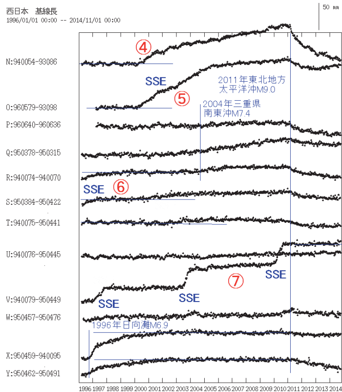
第2図(b) 基線長変化 (1996年から2014年10月) .
