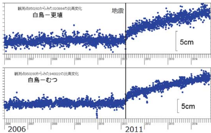
第5図 比高変化（2006年1月から2014年10月）. Fig. 5 Relative height changes between selected stations.
