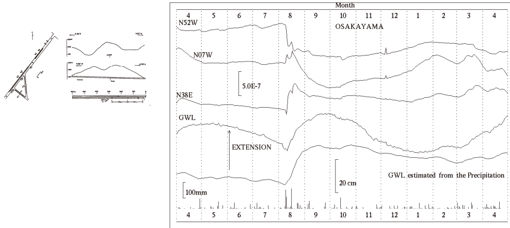
第5図 a 逢坂山観測所における歪変化と日雨量 (2014年4月～2015年4月) Fig.5a Strain change, underground water level and daily precipitation at Osakayama observatory. (Apr.01,2014～Apr.30,2015).
