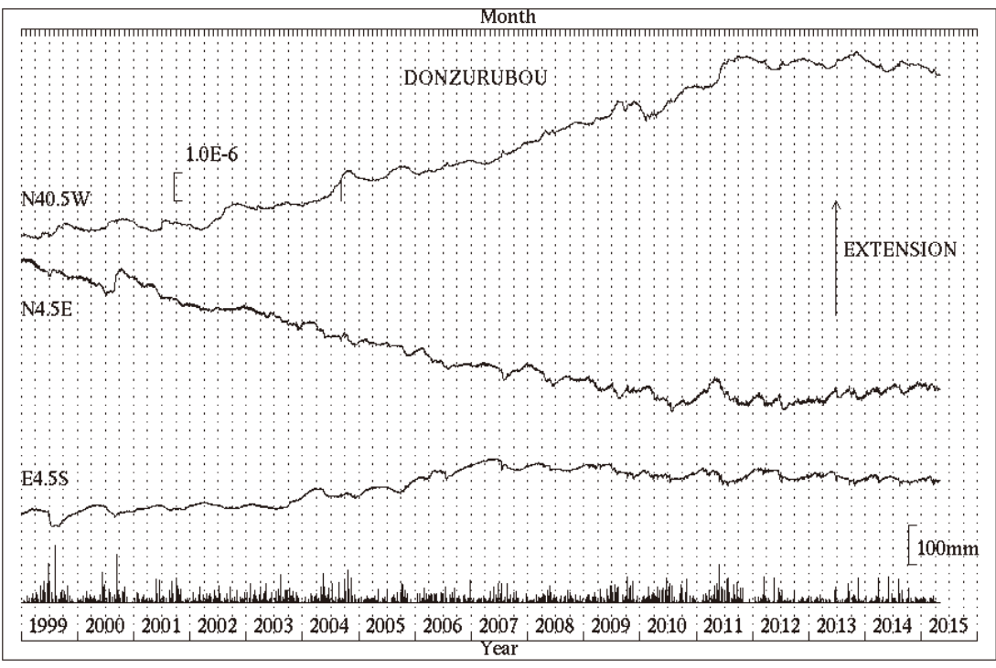
第4図 b 屯鶴峯観測所における歪変化と日雨量 (1999年1月~2015年4月) Fig.4b Strain changes and daily precipitation at Donzurubo observatory. (Jan. 1,1999 ~ Apr.30.,2015).
