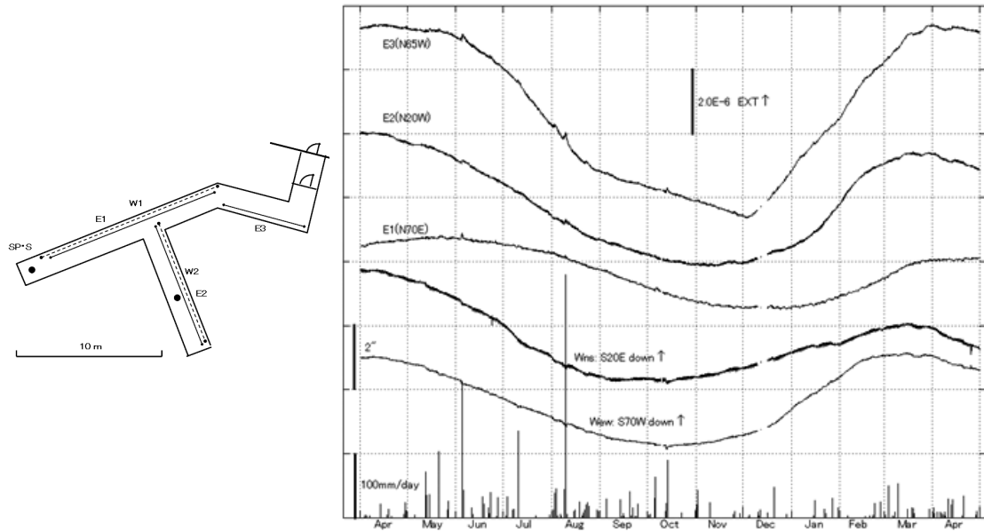
第8図 宿毛観測所における歪変化と日雨量 (2014年4月～2015年4月) Fig.8 Strain changes, tilt changes and daily precipitation at Sukumo station. (Apr.01, 2014～Apr.30,2015).
