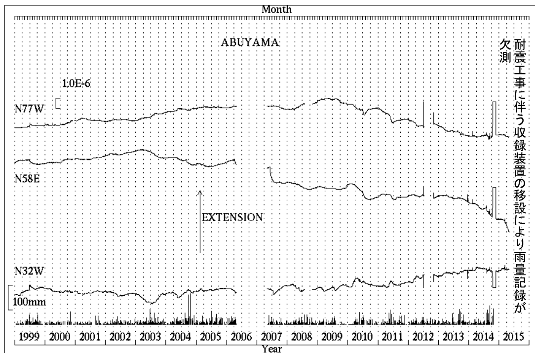
第3図 b 阿武山観測所における歪変化と日雨量（1999年1月～2015年4月） Fig.3b Strain changes and daily precipitation at Abuyama observatory. (Jan. 1,1999 ~ Apr.30,2015).
