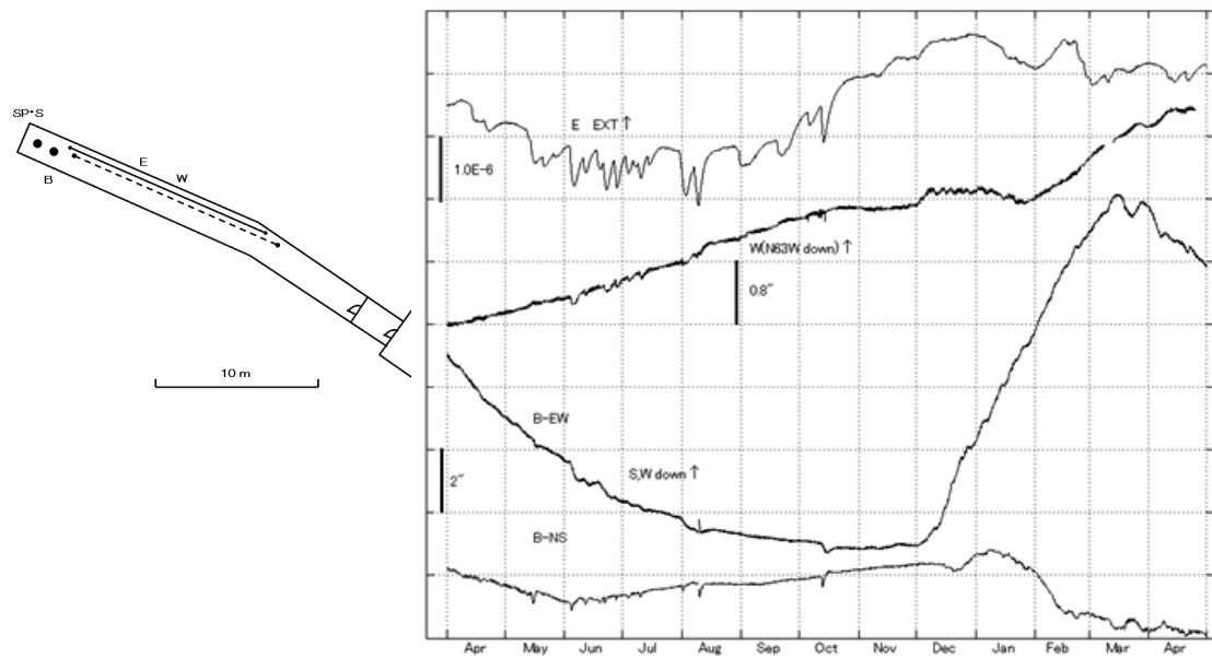
第9図 高城観測所における歪変化と傾斜変化 (2014年4月～2015年4月) Fig.9 Strain changes and tilt changes at Takajo station. (Apr.01, 2014～Apr.30,2015).
