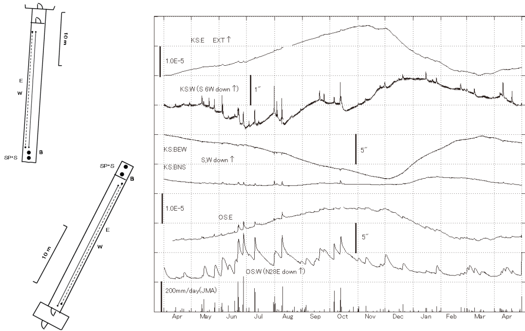
第 10 図 串間・大隈観測所における歪・傾斜変化 (2014 年 4 月～2015 年 4 月) Fig.10 Strain changes and tilt changes at Kushima, and Ohsumi station. Lowest bar graph is daily precipitation at Tashiro, nearest station by JMA. (Apr.01, 2014～Apr.30,2015).
