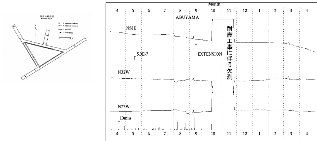
第3図 a 阿武山観測所における歪変化と日雨量（2014年4月～2015年4月） Fig.3a Strain changes and daily precipitation at Abuyama observatory. (Apr.01,2014～Apr.30,2015).
