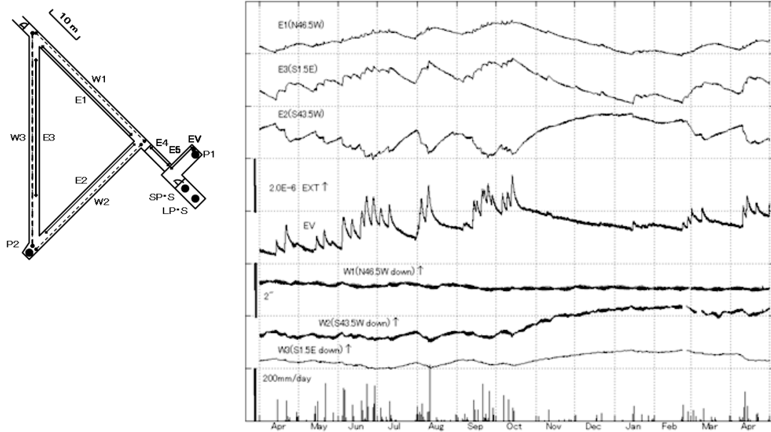
第6図 宮崎観測所における歪・傾斜変化と日雨量 (2014年4月~2015年4月) Fig.6 Strain changes, tilt changes and daily precipitation at Miyazaki observatory. (Apr.01, 2014~Apr.30,2015).
