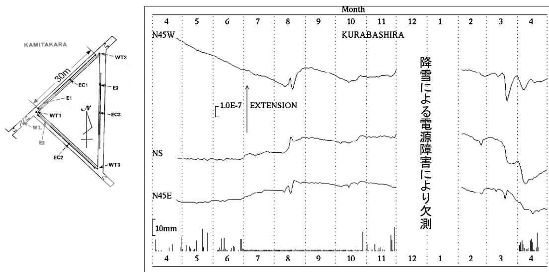
第 2 図 上宝観測所蔵柱観測室における歪変化と日雨量 (2014 年 4 月～2015 年 4 月)
