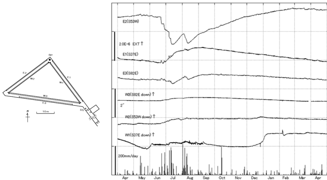
第7図 伊佐観測所における歪・傾斜変化と日雨量 (2014年4月~2015年4月) Fig.7 Strain changes, tilt changes and daily precipitation at Isa station. (Apr.01, 2014~Apr.30,2015).
