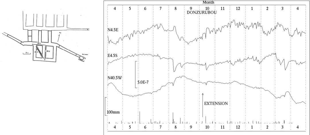
第4図 a 屯鶴峯観測所における歪変化と日雨量 (2014年4月~2015年4月) Fig.4a Strain changes and daily precipitation at Donzurubo observatory. (Apr.01,2014~Apr.30,2015).
