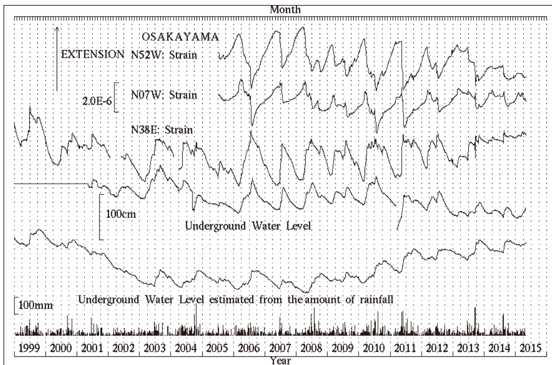
第5図 b 逢坂山観測所における歪変化と日雨量 (1999年1月～2015年4月) Fig.5b Strain change, underground water level, daily precipitation and estimated underground water level from precipitation at Osakayama observatory. (Jan. 1,1999 ~ Apr.30,2015).
