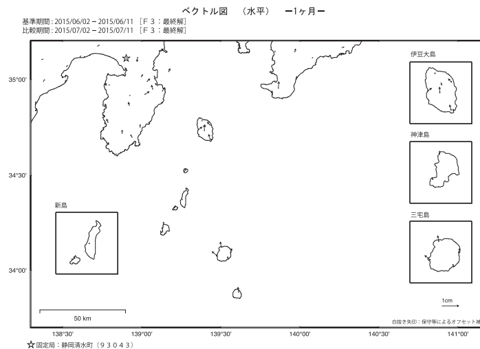
第2図a GNSS観測による伊豆地方の水平変動 (1ヶ月) Fig. 2a Horizontal movements of Izu Region by GNSS continuous measurements (1 month).
