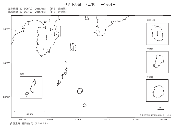
第2図b GNSS観測による伊豆地方の上下変動 (1ヶ月) Fig. 2b Vertical movements of Izu Region by GNSS continuous measurements (1 month).
