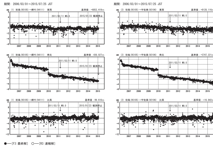
第3図b 伊豆半島東部GNSS連続観測結果(2006年3月以降・3成分)
