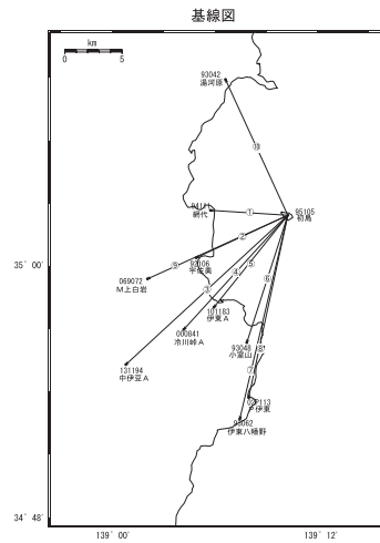
第3図a 伊豆半島東部GNSS連続観測結果(基線図)
