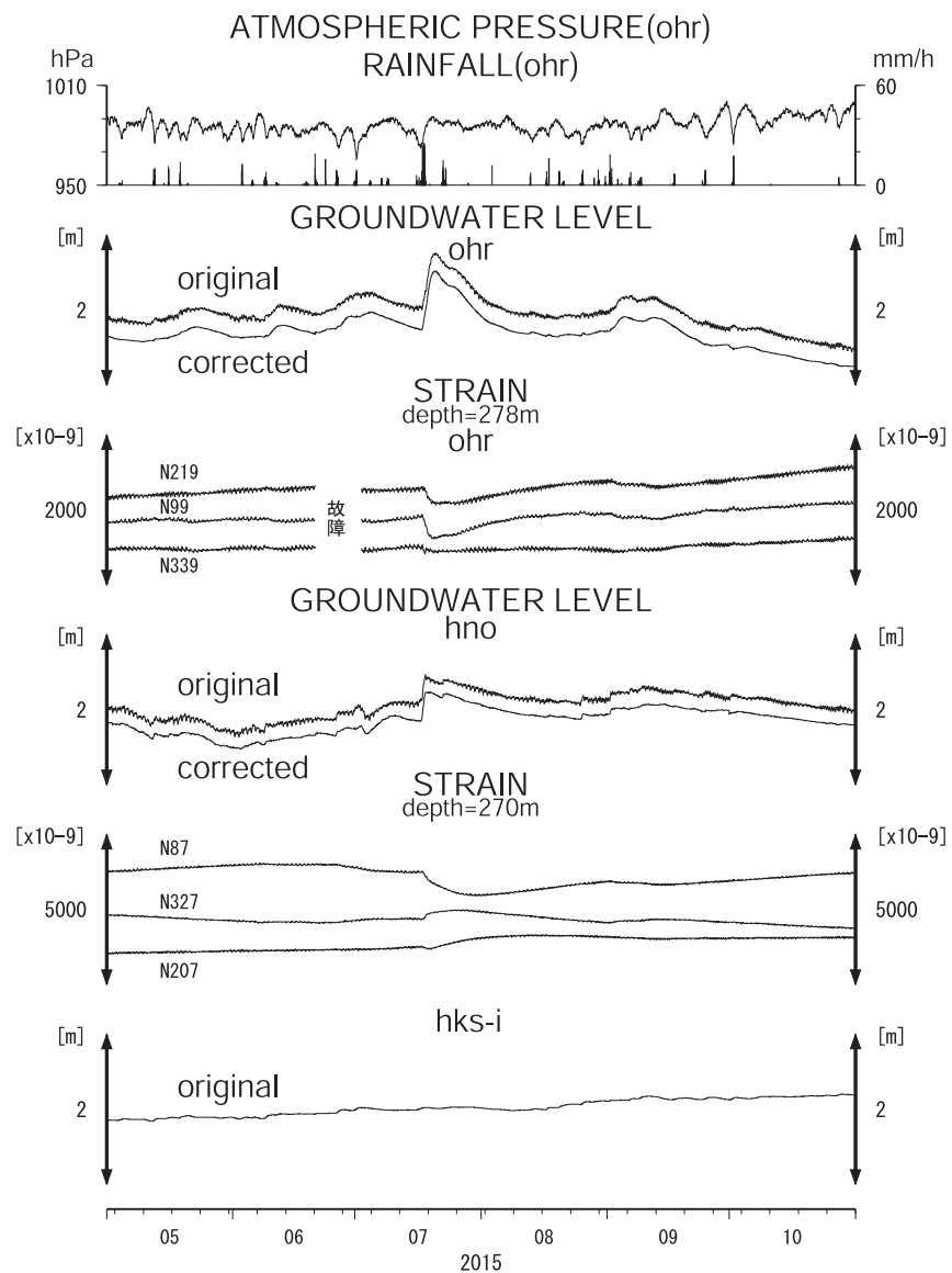
第5図 ohr, hno, hks-iの地下水位・地殻歪の2015年5月～2015年10月の観測結果.
