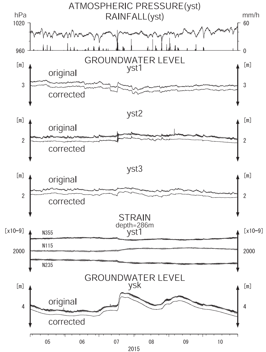
第2図 yst1, yst2, yst3, ysk の2015年5月~2015年10月の観測結果. Fig.2 Observation results at yst1, yst2, yst3 and ysk from May 2015 to October 2015.
