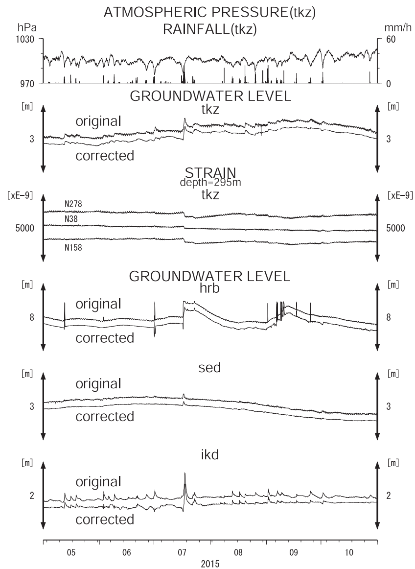
第3図 tkz,hrb,sed,ikdの2015年5月～2015年10月の観測結果。 Fig.3 Observation results at tkz, hrb, sed and ikd from May 2015 to October 2015.
