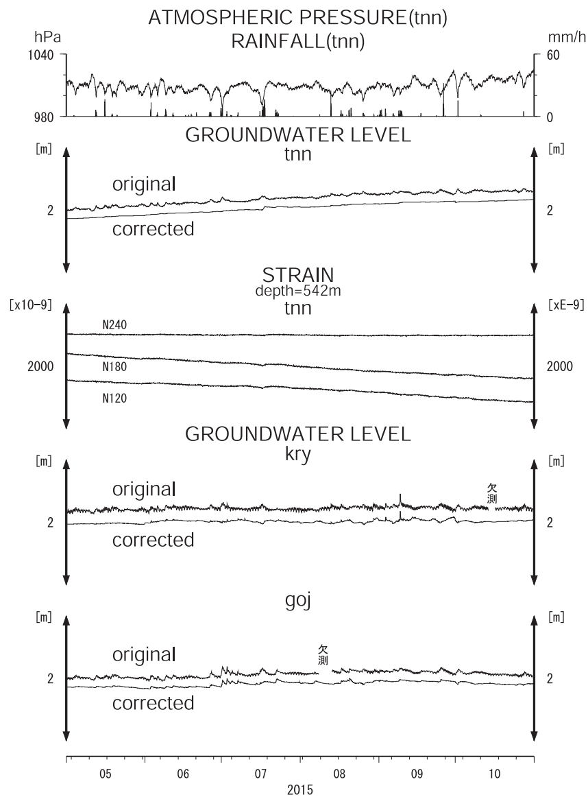
第4図 tnn,kry,gojの2015年5月～2015年10月の観測結果。 Fig.4 Observation results at tnn, kry and goj from May 2015 to October 2015.
