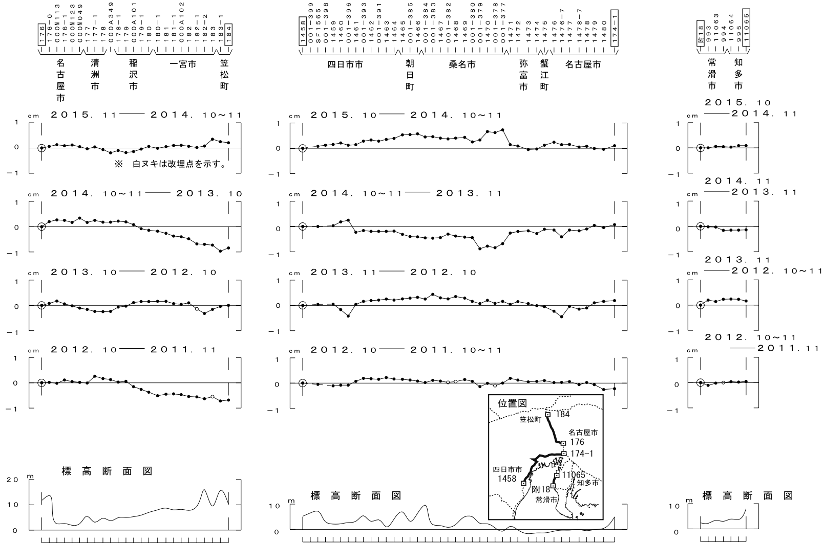
第1図 中京の上下変動 Fig.1 Results of leveling survey around Nagoya city.
