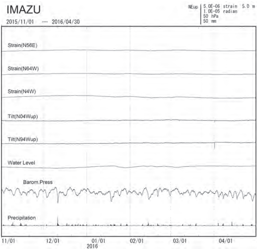
第2図 今津観測点における(上)2013年5月～2016年4月,(下)2015年11月～2016年4月のひずみ・傾斜変化(時間値)。毎年冬のひずみ・水位変化は、観測点付近の融雪のための地下水汲み上げに伴うもの。
