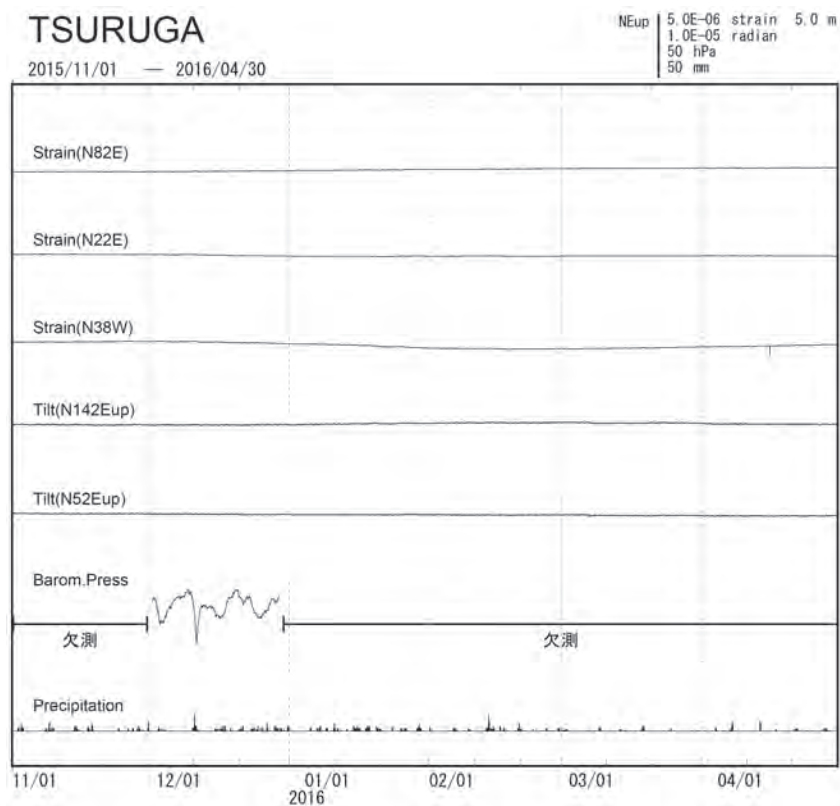
第3図 敦賀観測点における(上)2013年5月～2016年4月、(下)2015年11月～2016年4月のひずみ・傾斜変化(時間値)。
