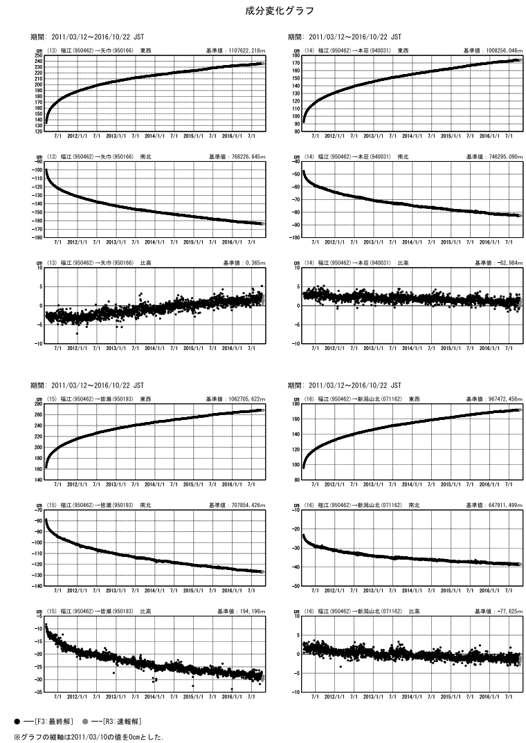
第10図 東北地方太平洋沖地震後の地殻変動 Fig. 10 Crustal deformation after the 2011 off the Pacific coast of Tohoku Earthquake (4/5).
