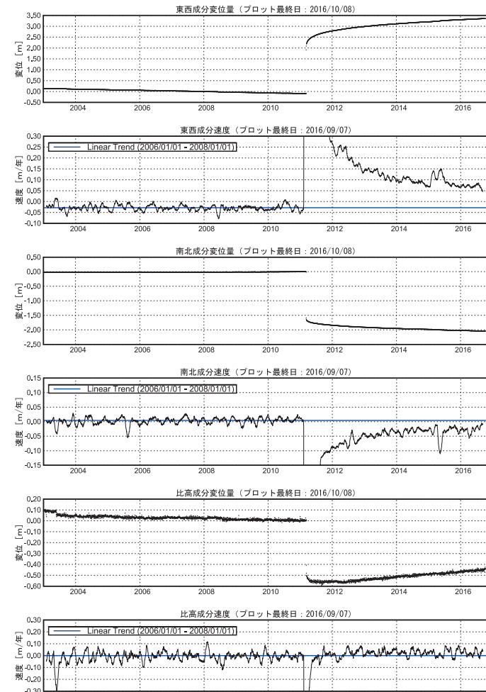
第 13 図 東北地方太平洋岸の GEONET 観測点における地殻変動速度 の変化（山田観測点・時系列）
