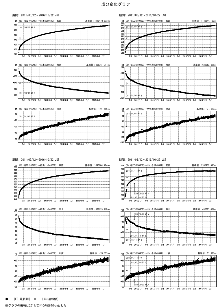
第8図 東北地方太平洋沖地震後の地殻変動 Fig. 8 Crustal deformation after the 2011 off the Pacific coast of Tohoku Earthquake (2/5).
