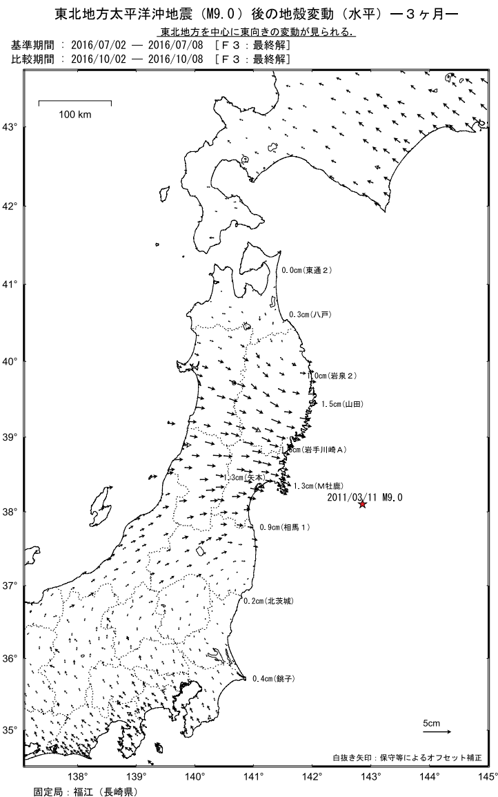
第4図 2011年東北地方太平洋沖地震後の地殻変動 (最近3ヶ月、水平) Fig. 4 Crustal deformation after the 2011 off the Pacific coast of Tohoku Earthquake (three months , horizontal displacement).
