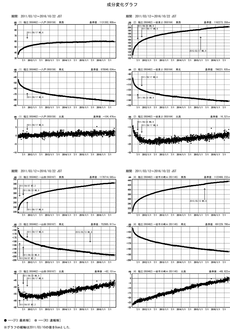
第7図 東北地方太平洋沖地震後の地殻変動 Fig. 7 Crustal deformation after the 2011 off the Pacific coast of Tohoku Earthquake (1/5).
