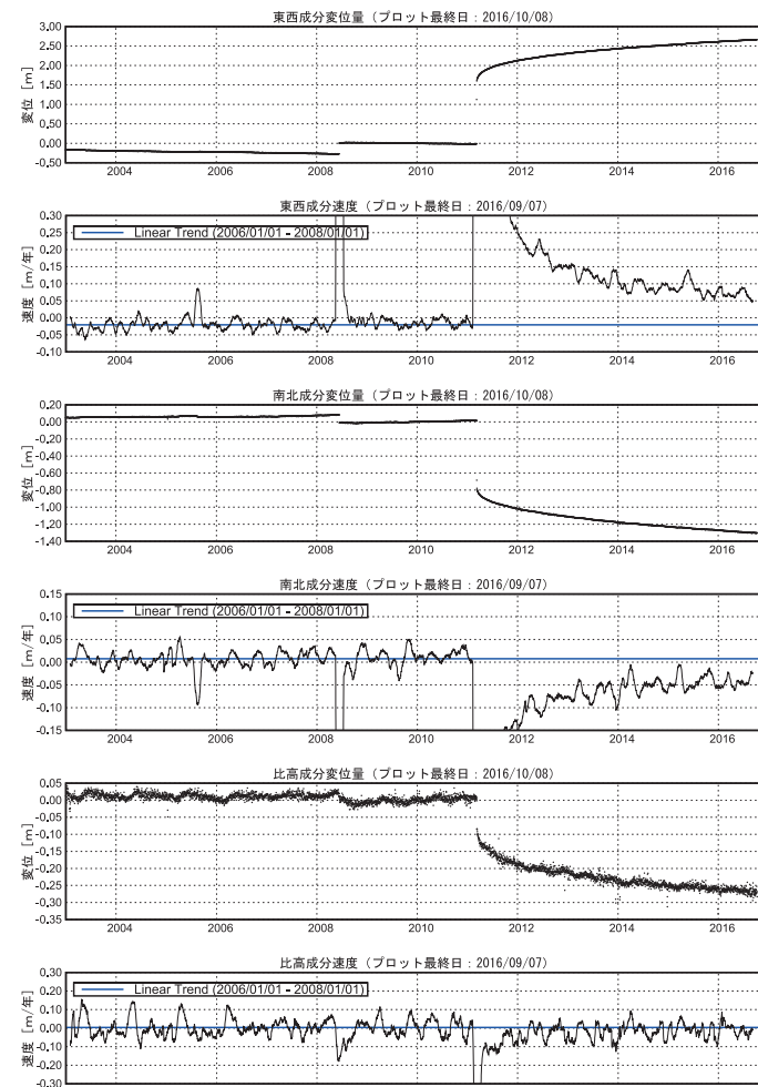
第 17 図 東北地方太平洋岸の GEONET 観測点における地殻変動速度 の変化（皆瀬観測点・時系列）
