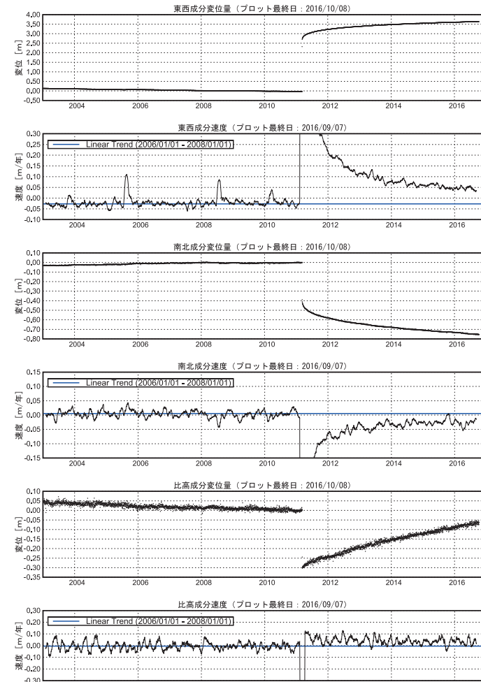
平成23年(2011年)東北地方太平洋沖地震前後の地殻変動 東北地方太平洋沖地震発生前の変動速度には戻っていない 三隅 (950388) -- 相馬 1 (940038) 間の成分変位と速度グラフ
