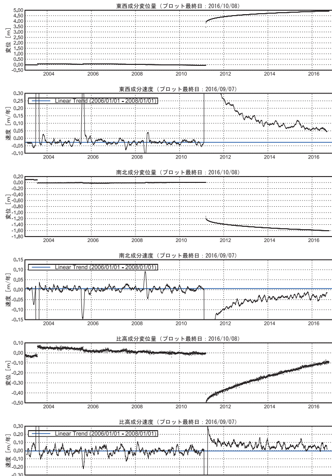
平成23年(2011年)東北地方太平洋沖地震前後の地殻変動 東北地方太平洋沖地震発生前の変動速度には戻っていない 2015年5月13日に発生した宮城県沖の地震に伴う地殻変動の影響が見られる 三隅 (950388) -- 矢本 (960549) 間の成分変位と速度グラフ
