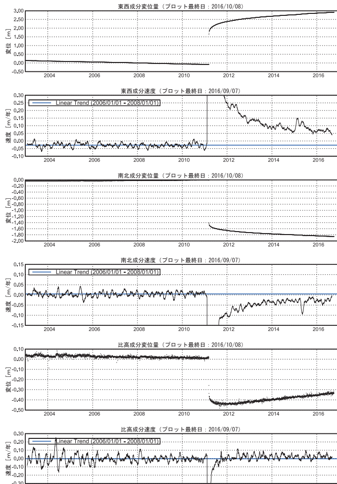
第 12 図 東北地方太平洋岸の GEONET 観測点における地殻変動速度 の変化（宮古観測点・時系列）
