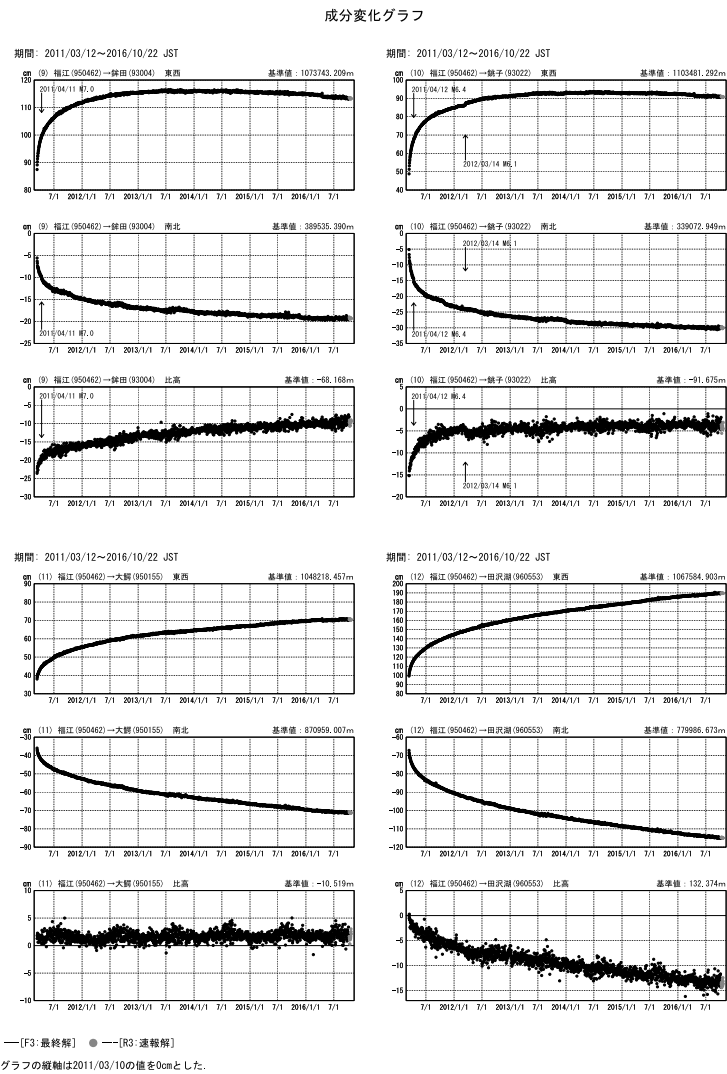
第9図 東北地方太平洋沖地震後の地殻変動 Fig. 9 Crustal deformation after the 2011 off the Pacific coast of Tohoku Earthquake (3/5).
