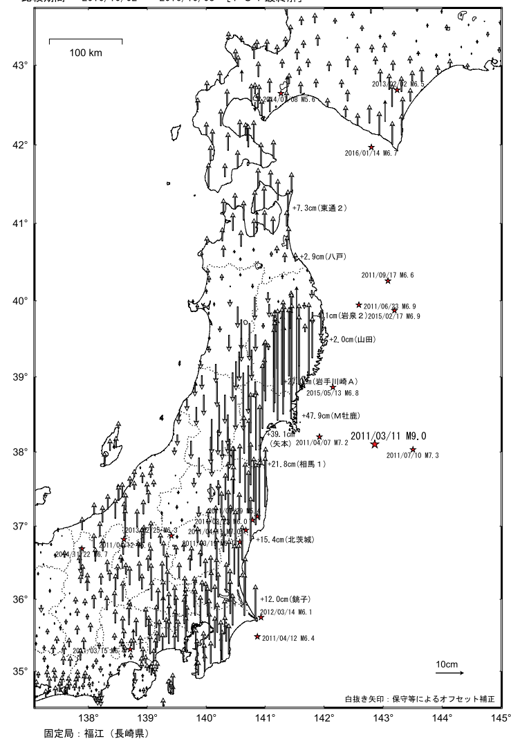
第2図 2011年東北地方太平洋沖地震後の累積地殻変動（上下） Fig. 2 Accumulated crustal deformation after the 2011 off the Pacific coast of Tohoku Earthquake (vertical).
