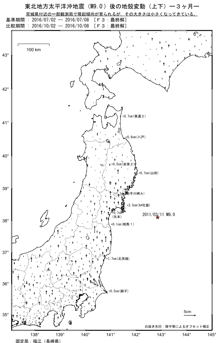
第5図 2011年東北地方太平洋沖地震後の地殻変動 (最近3ヶ月、上下) Fig. 5 Crustal deformation after the 2011 off the Pacific coast of Tohoku Earthquake (three months , vertical displacement).
