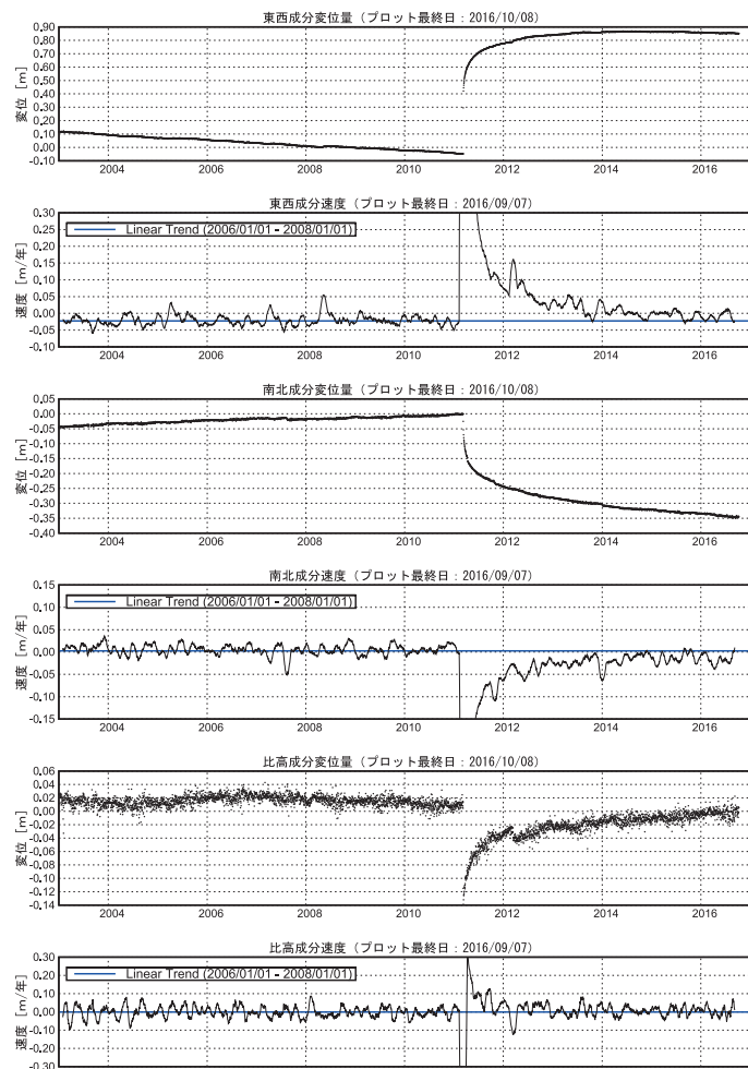
第 16 図 東北地方太平洋岸の GEONET 観測点における地殻変動速度 の変化（銚子観測点・時系列）
