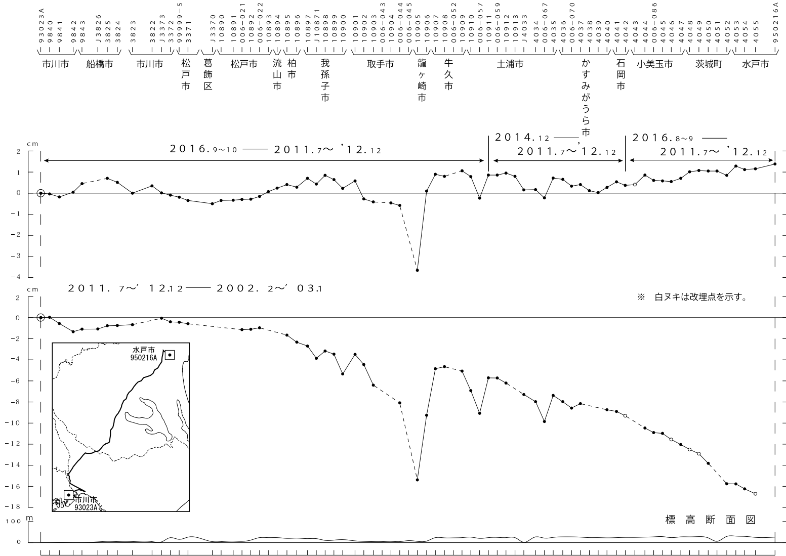
第1図 市川市～水戸市間の上下変動 Fig. 1 Results of leveling survey from Ichikawa city to Mito city.
