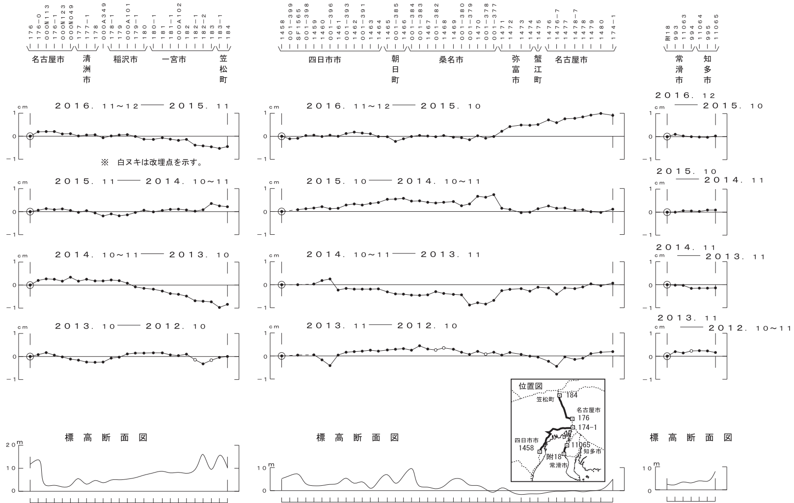
第1図 中京の上下変動 Fig.1 Results of leveling survey around Nagoya city.
