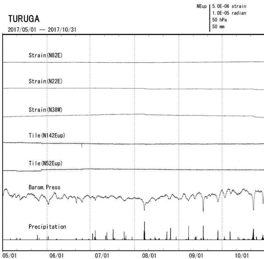
第 3 図 敦賀観測点における(上) 2014 年 11 月～2017 年 10 月, (下 d)2017 年 5 月～2017 年 10 月のひずみ・傾斜変化 (時間値).
