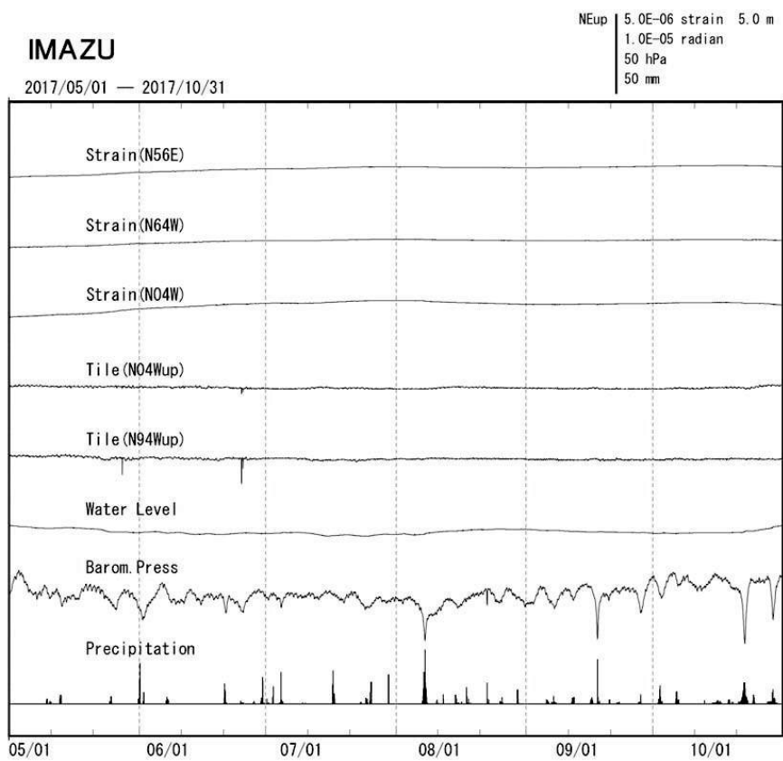
第2図 今津観測点における(上) 2014年11月～2017年10月、(下)2017年5月～2017年10月のひずみ・傾斜変化(時間値)。毎年冬のひずみ・水位変化は、観測点付近の融雪のための地下水汲み上げに伴うもの。
