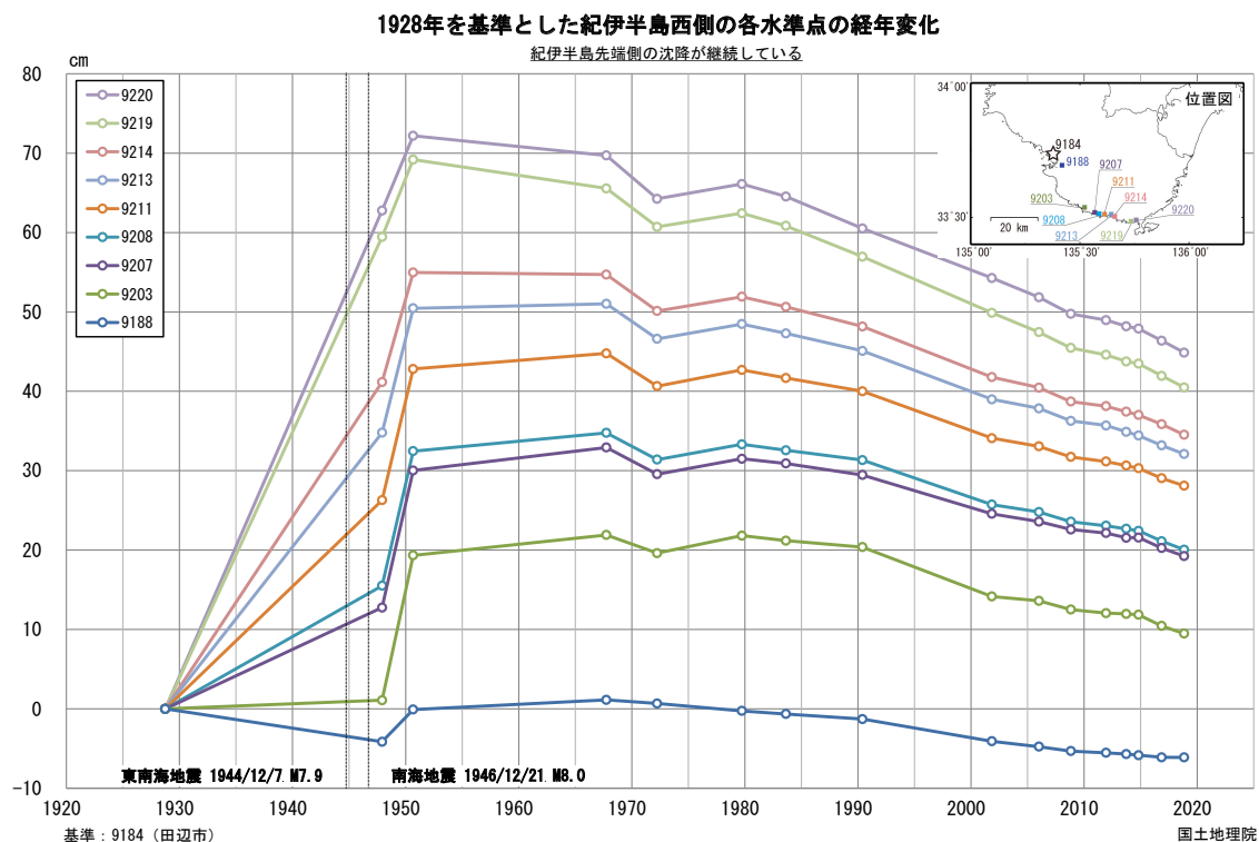
第9図 水準点9184（田辺市）を基準とした紀伊半島西側の各水準点の高さの上下変動時系列 Fig. 9 Time series of height changes of benchmarks along the leveling route on the coast of western Kii Peninsula from BM9184 (Tanabe) to BM9220 (Kushimoto) referred to BM9184 (Tanabe).
