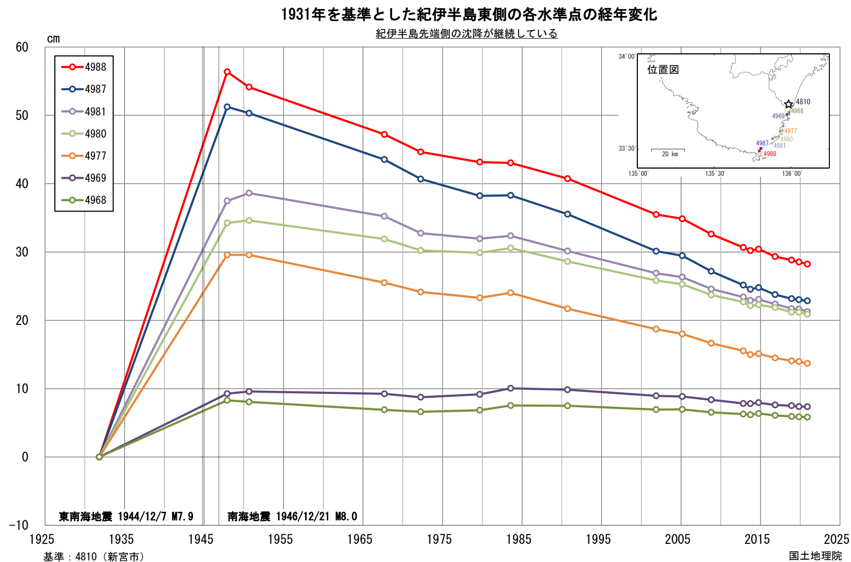
第 22 図 水準点 4810 (新宮市) を基準とした紀伊半島東側の各水準点の高さの上下変動時系列 Fig. 22 Time series of height changes of benchmarks along the leveling route on the east side of the Kii Peninsula referred to BM4810 (Shingu).
